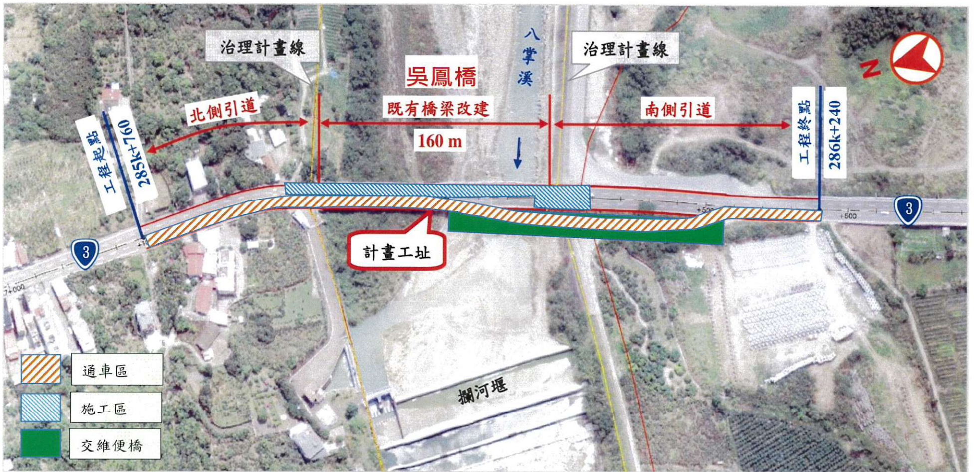
第 2-1 階段交通維持示意圖(北上線側橋梁及 A2 橋台拆除，部分南下線路段配合外側交維便橋通行)
