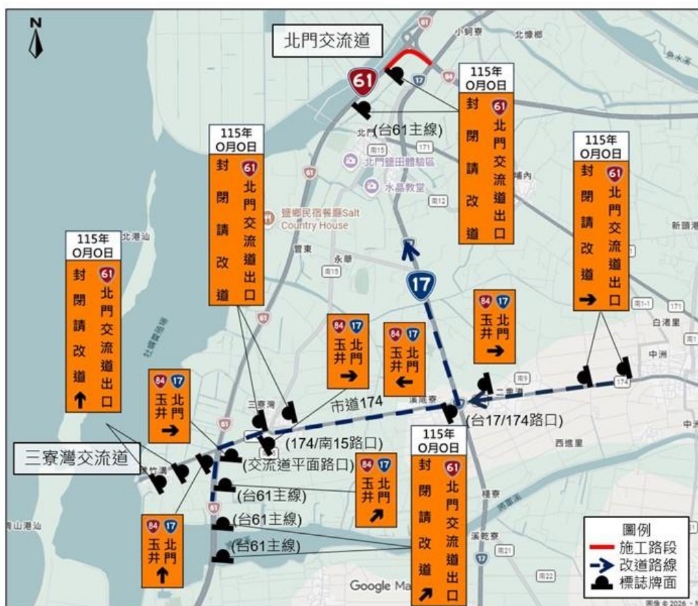
圖 4.2-5 台 61 線北上接台 17 線施工改道路線示意圖
