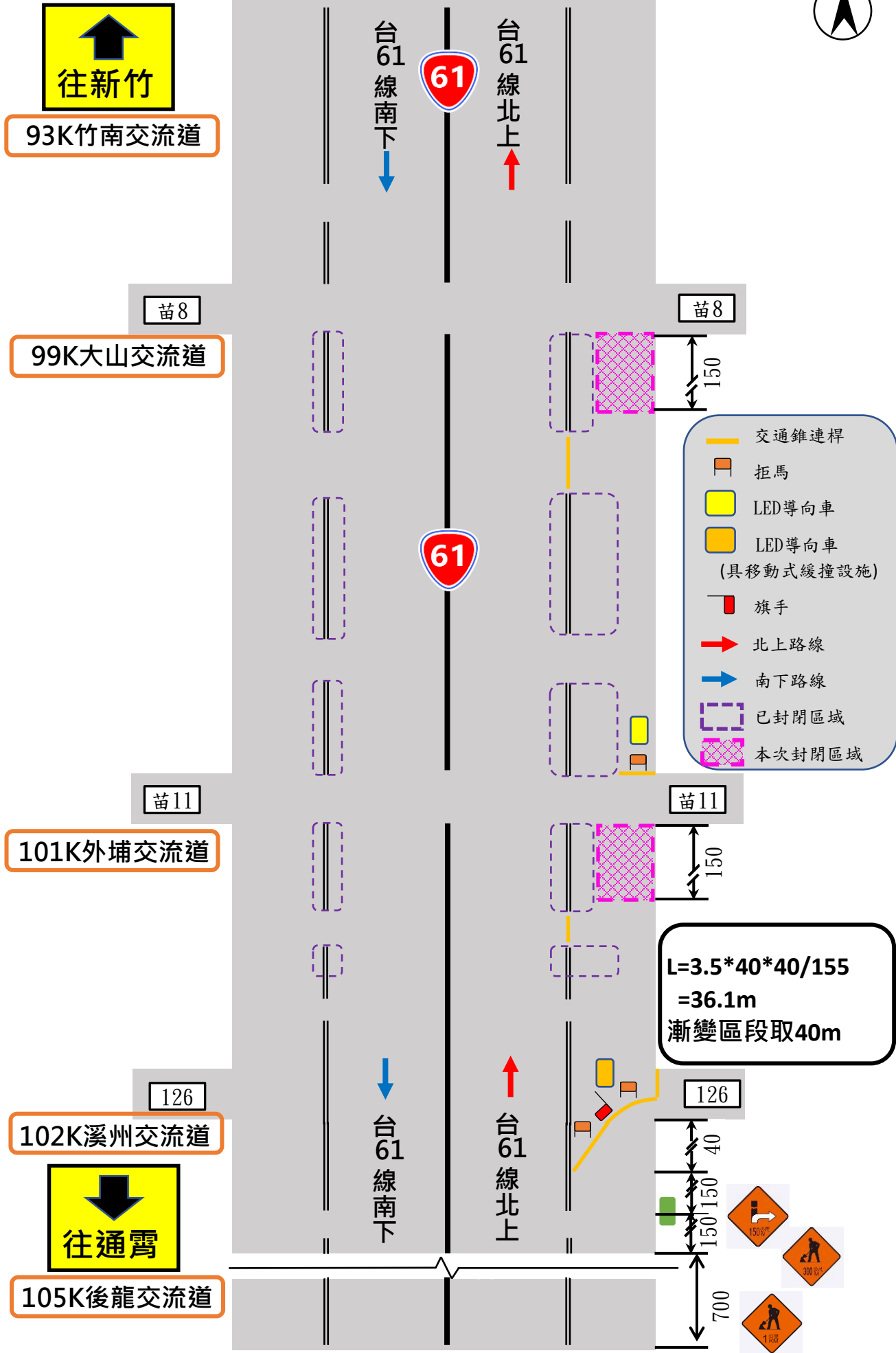
附件4 北上側車道交維佈設圖
