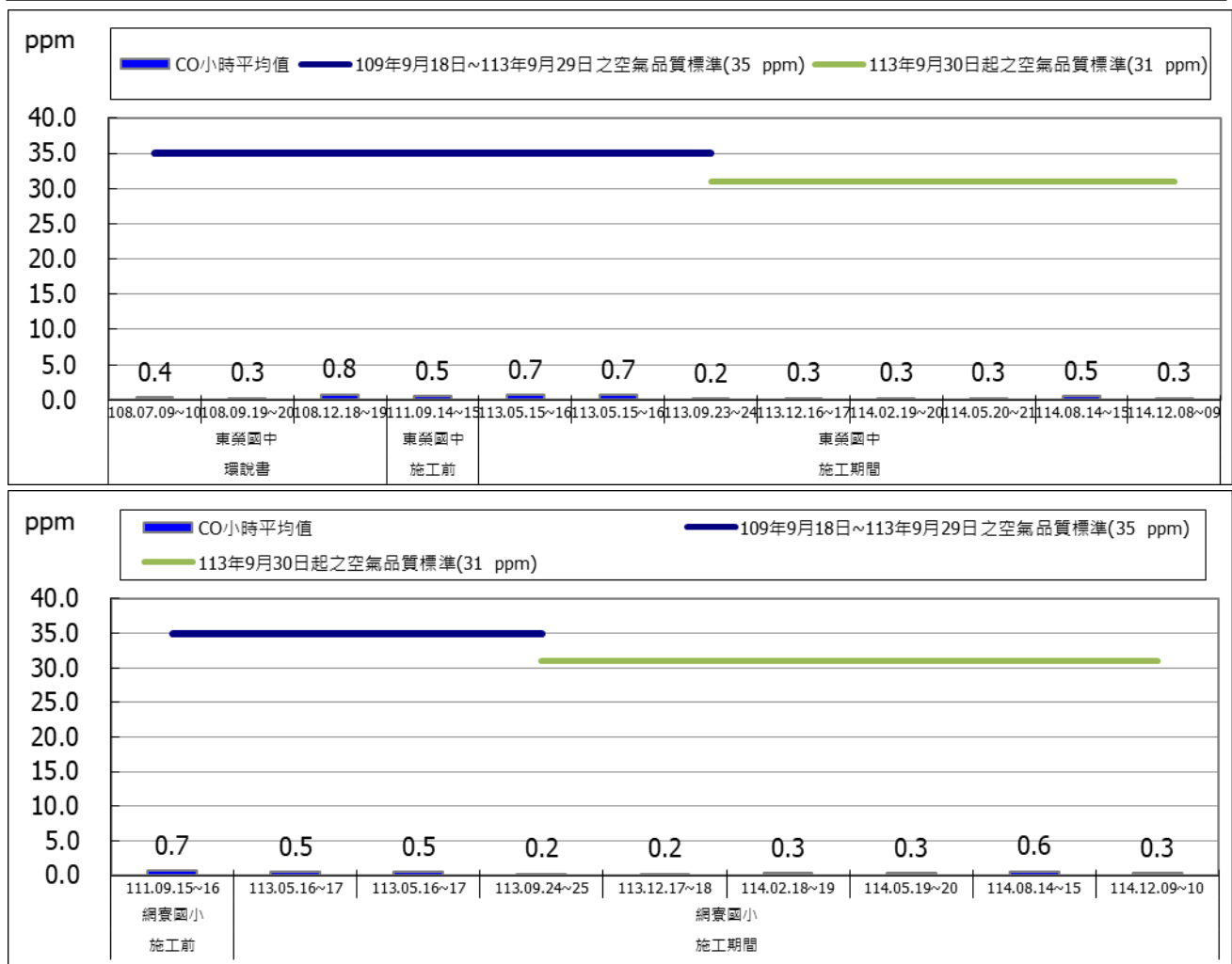
圖 2.1-12 一氧化碳(CO)測值小時平均值監測成果圖
