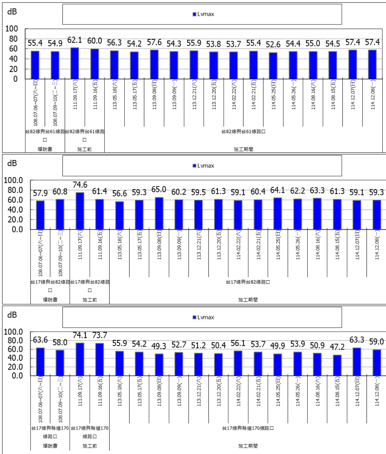
圖 2.2-9 各測站(L Vmax )環境振動監測成果圖
