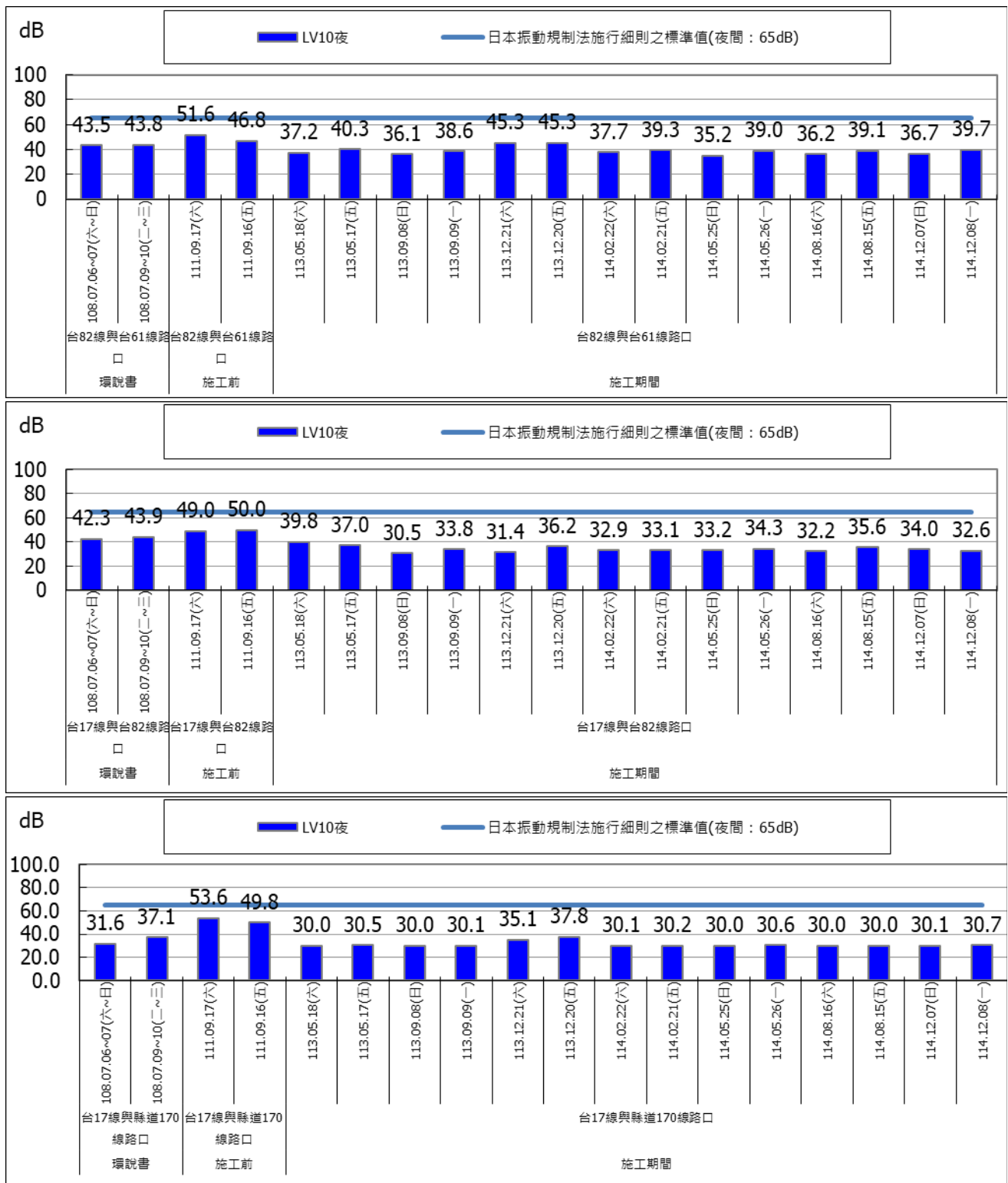
圖 2.2-8 各測站(LV10 夜)環境振動監測成果圖
