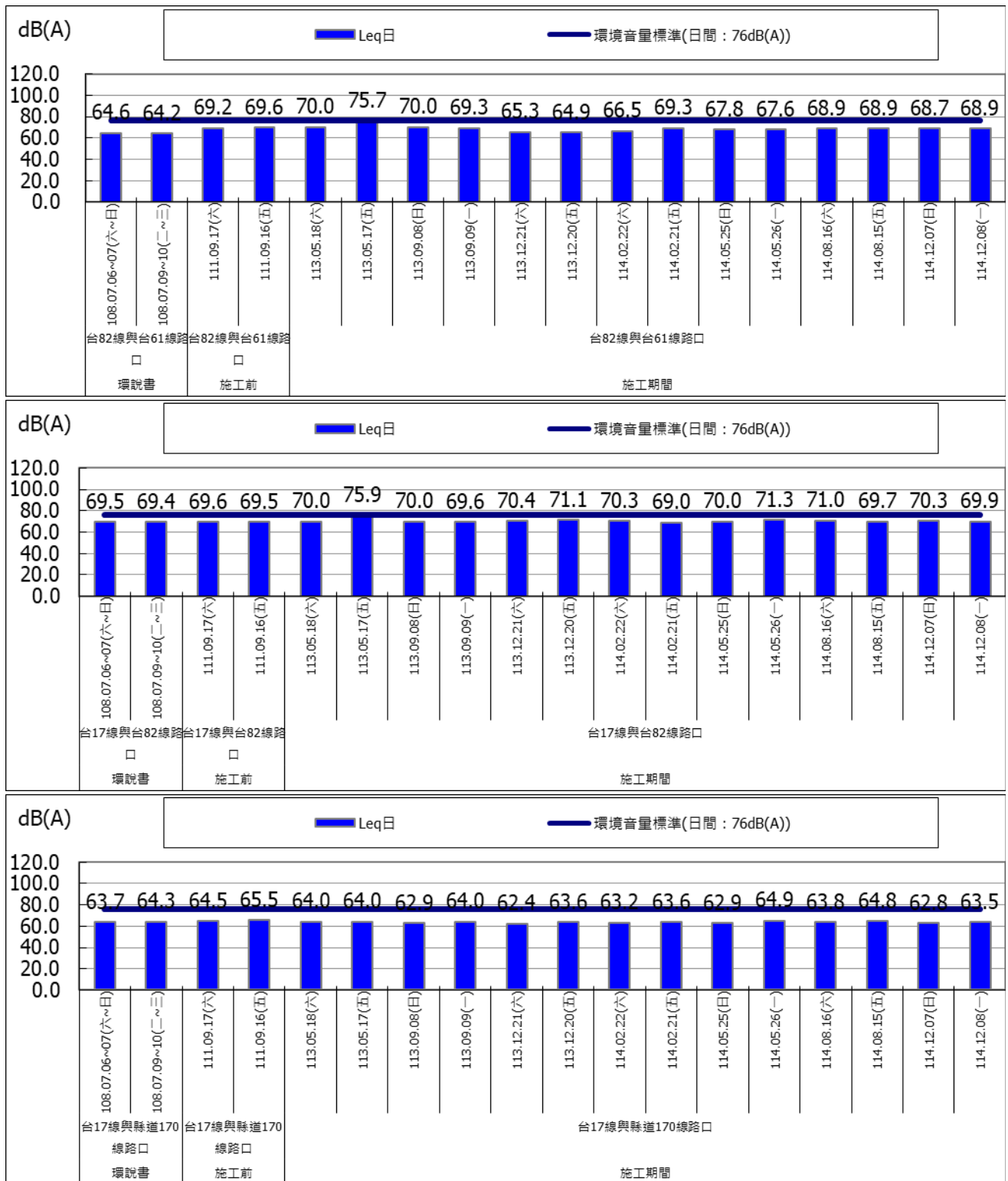
圖 2.2-1 各測站( L_{eq\text{日}} )環境噪音監測成果圖
