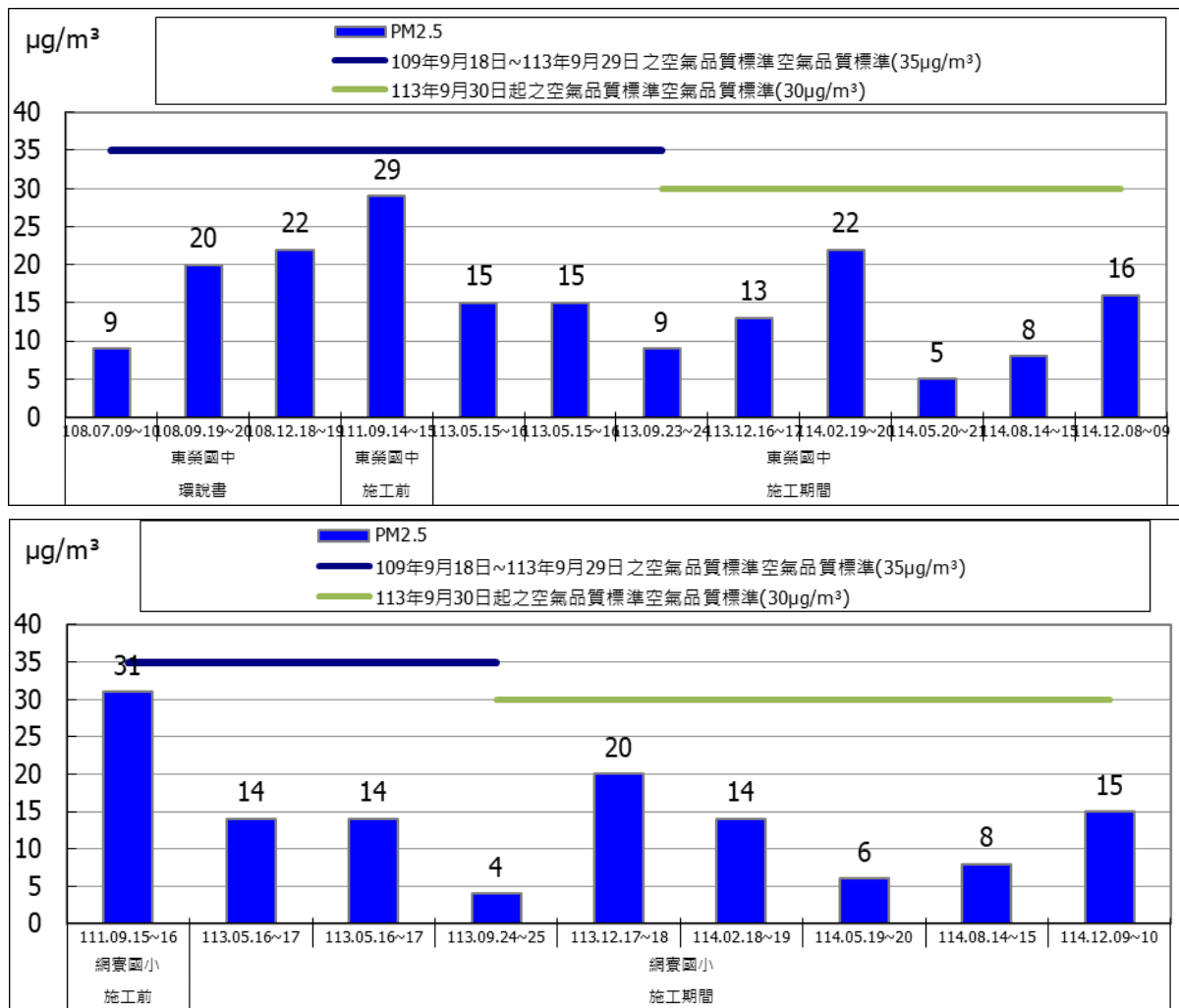
圖 2.1-2 懸浮微粒(PM 2.5 )測值 24 小時值監測成果圖
