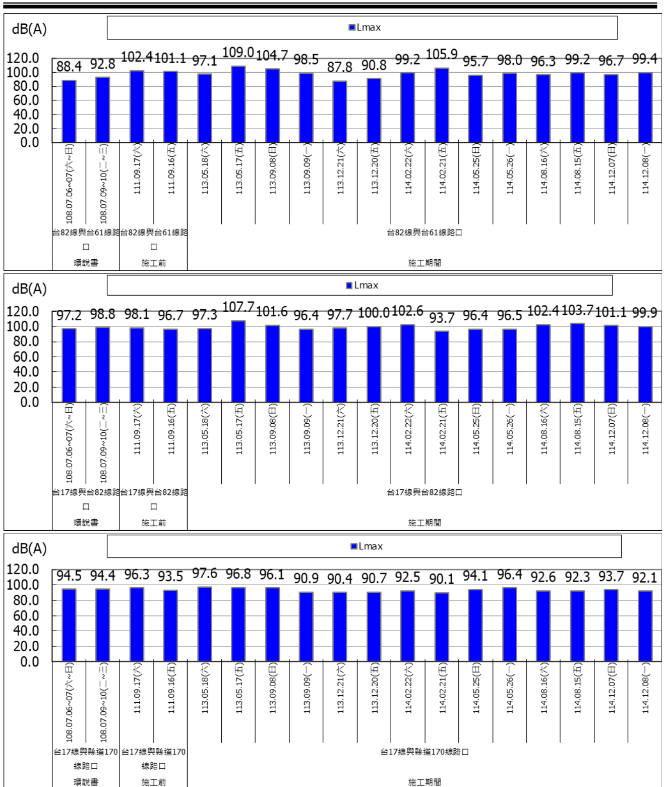
圖 2.2-4 各測站(L max )環境噪音監測成果圖
