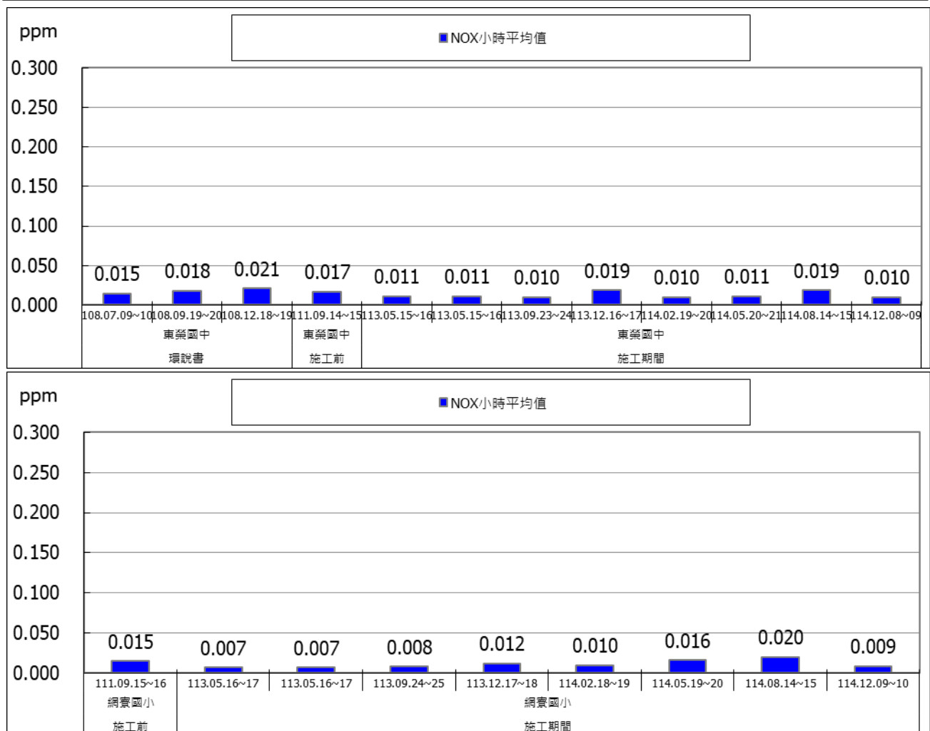
圖 2.1-8 氮氧化物(NO x )測值小時平均值監測成果圖
