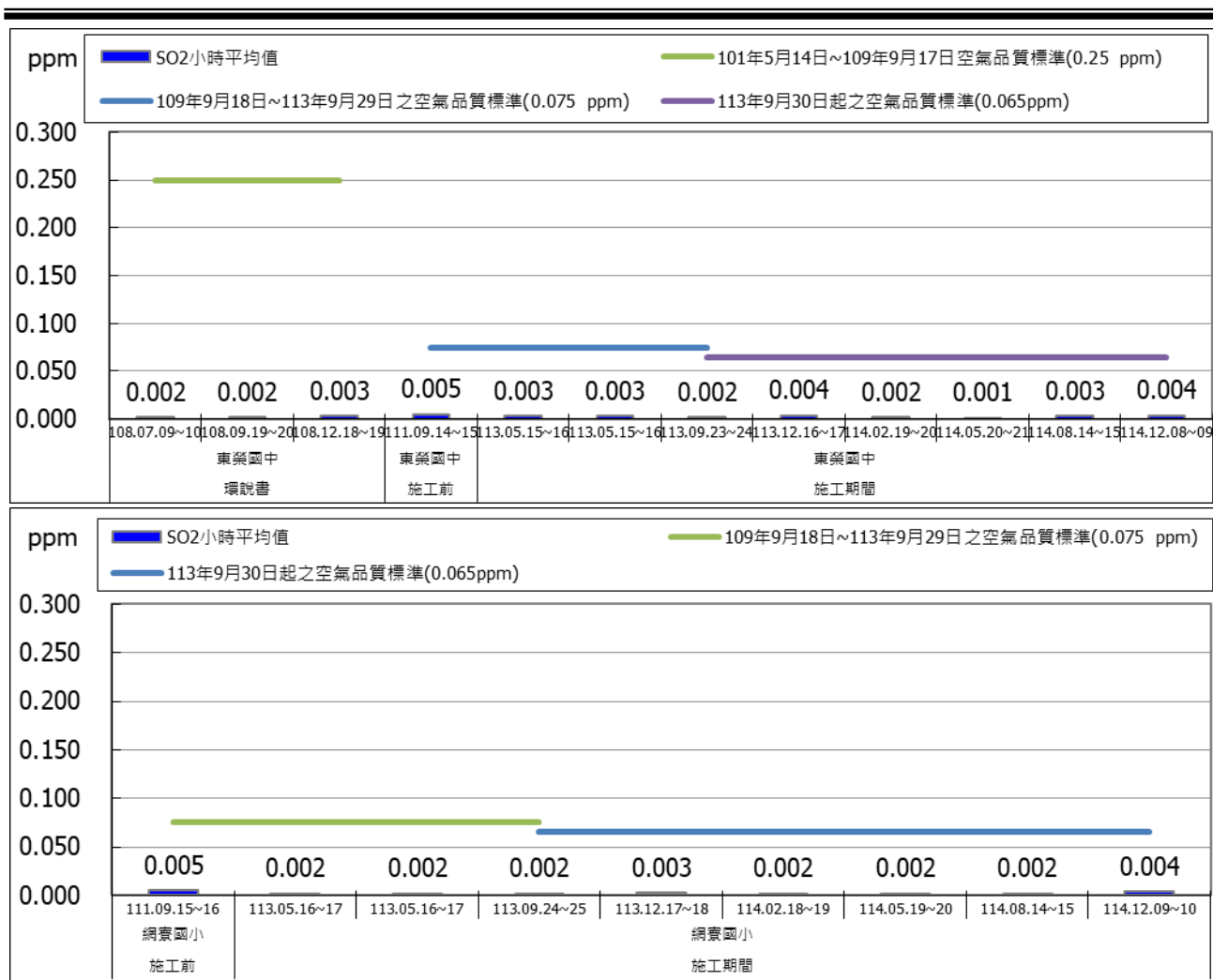
圖 2.1-10 二氧化硫(SO 2 )測值小時平均值監測成果圖
