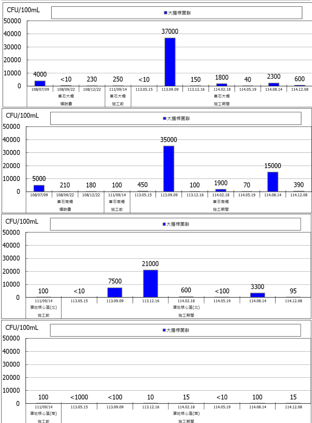
圖 2.3-10 地表水監測成果圖(大腸桿菌群)
