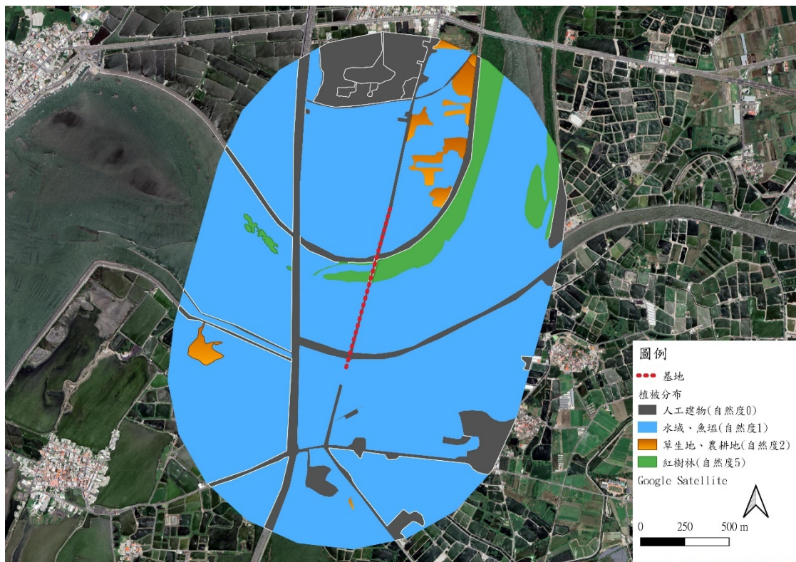
圖 2.5-1 植被及自然度分布圖(施工期間 114 年 7 月)
