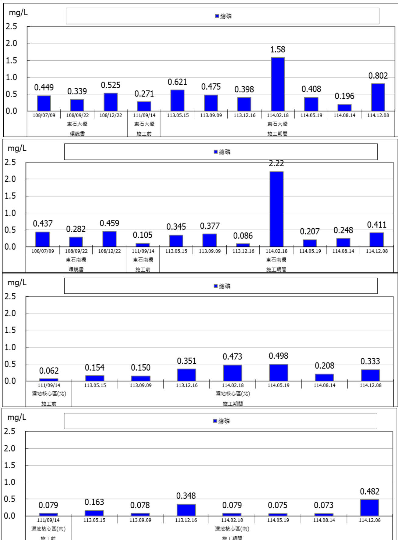
圖 2.3-9 地表水監測成果圖(總磷)
