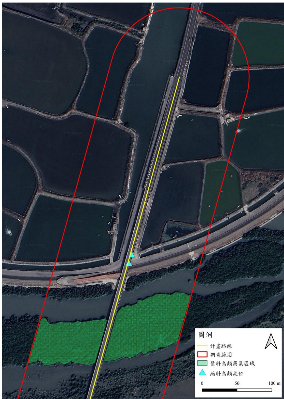
圖 2.7-2 鳥類築巢位置圖(施工期間 113 年 4 月)
