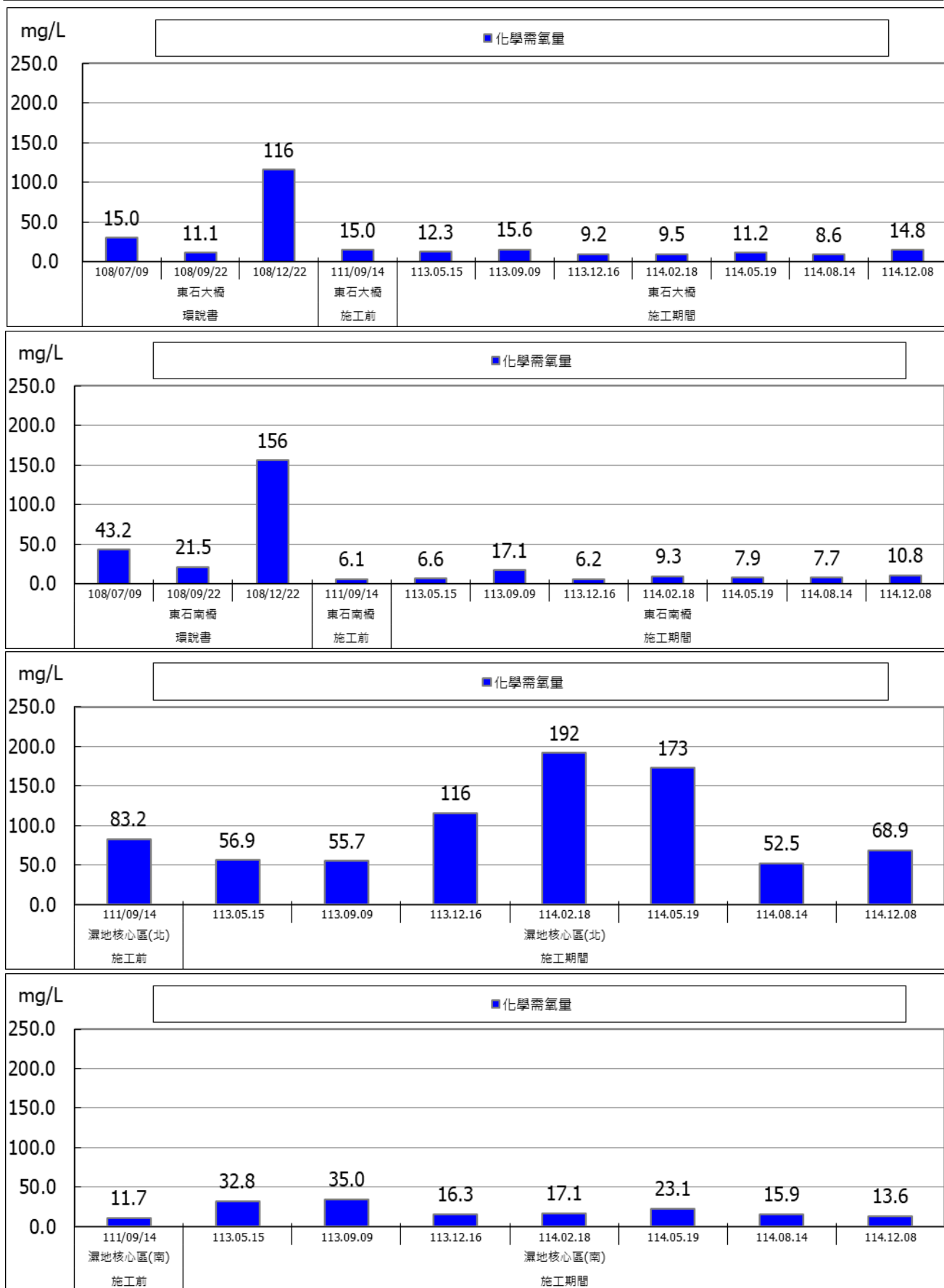
圖 2.3-5 地表水監測成果圖(化學需氧量)
