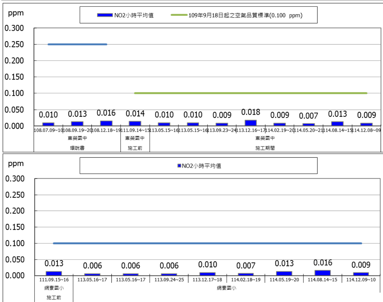
圖 2.1-6 二氧化氮(NO 2 )測值小時平均值監測成果圖
