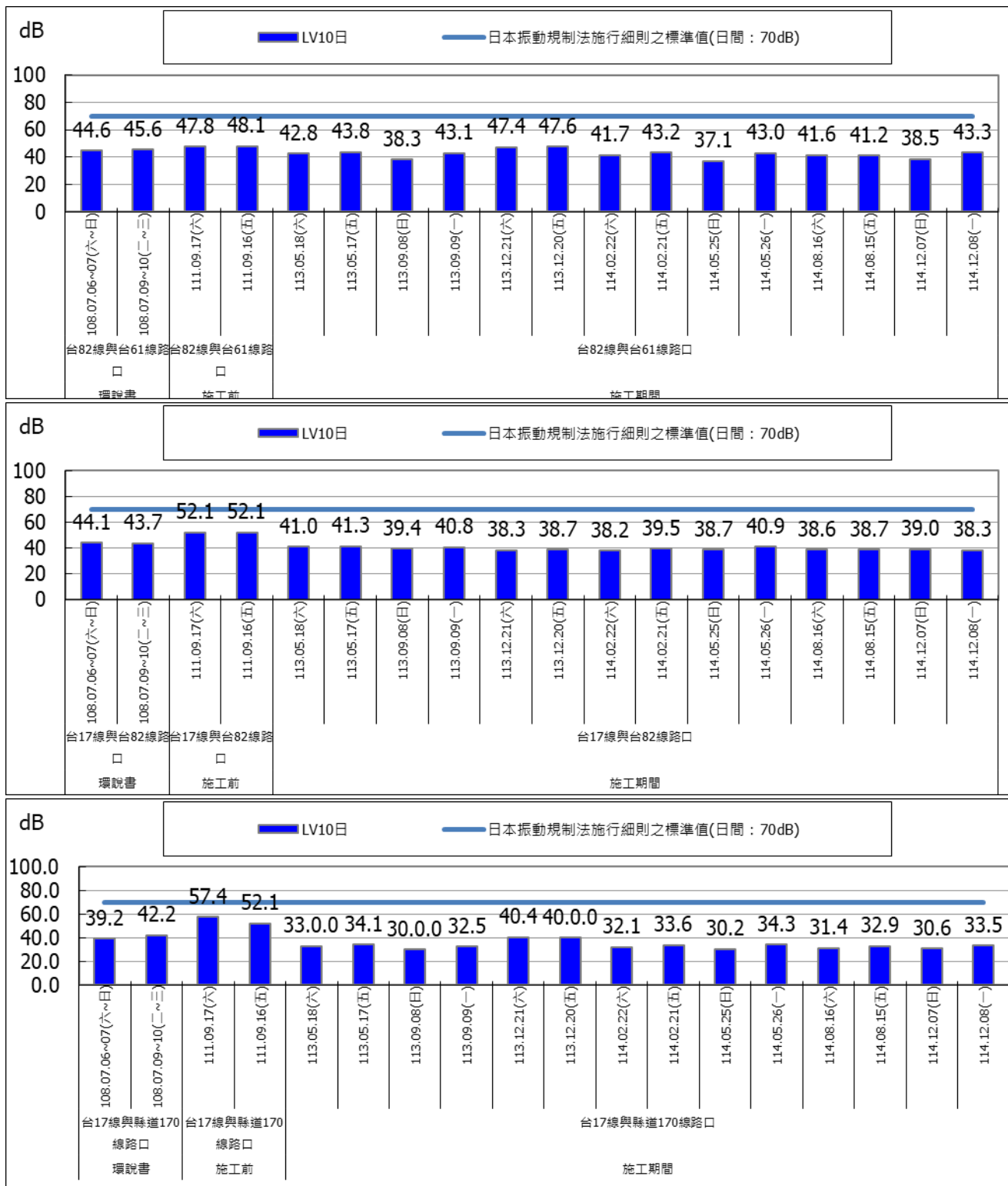
圖 2.2-7 各測站(LV10日)環境振動監測成果圖
