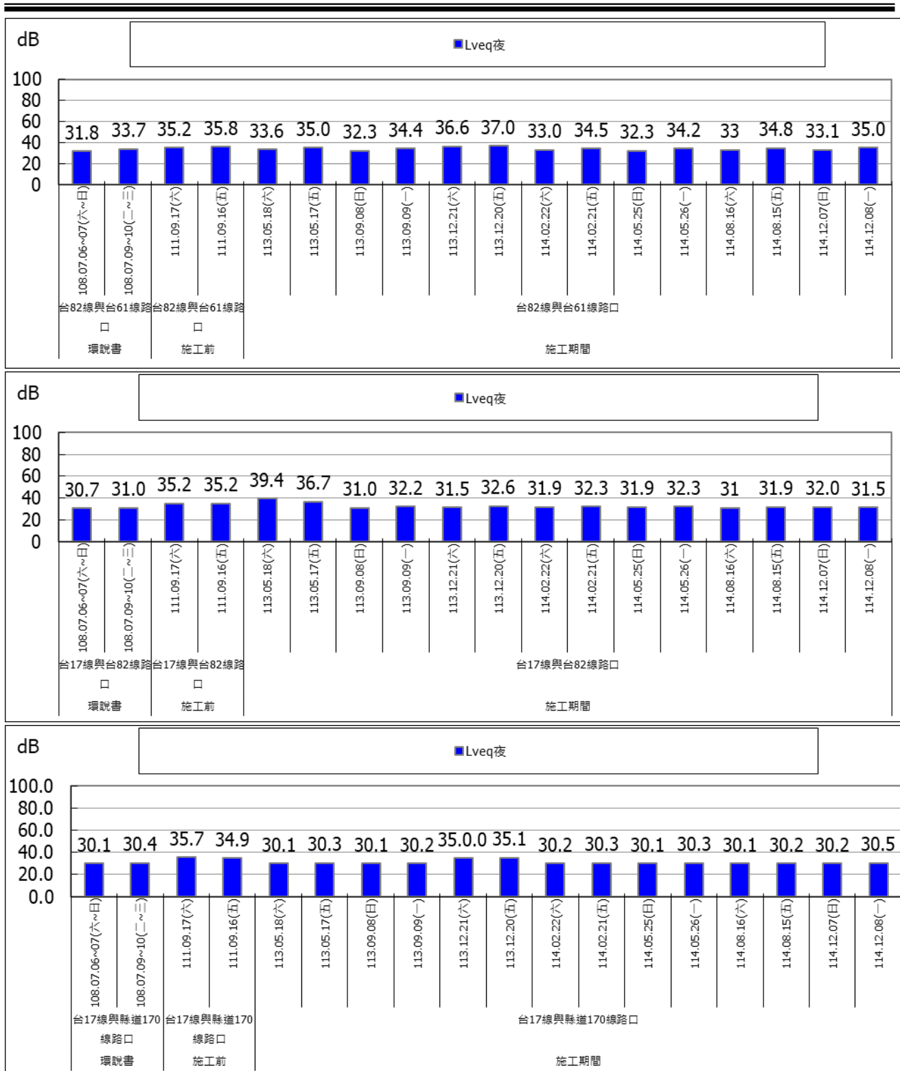
圖 2.2-6 各測站(L veq 夜)環境振動監測成果圖
