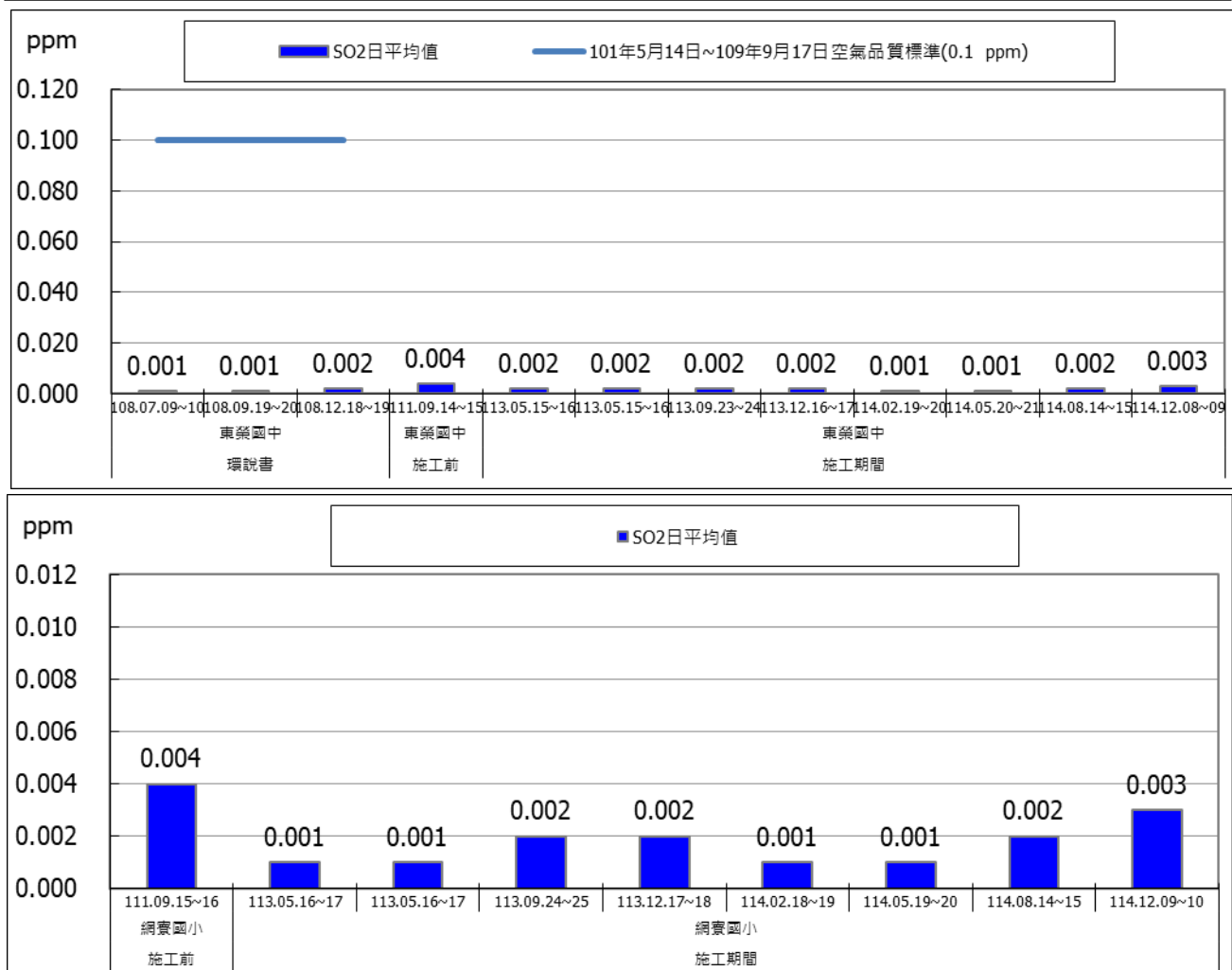
圖 2.1-9 二氧化硫(SO 2 )測值日平均值監測成果圖
