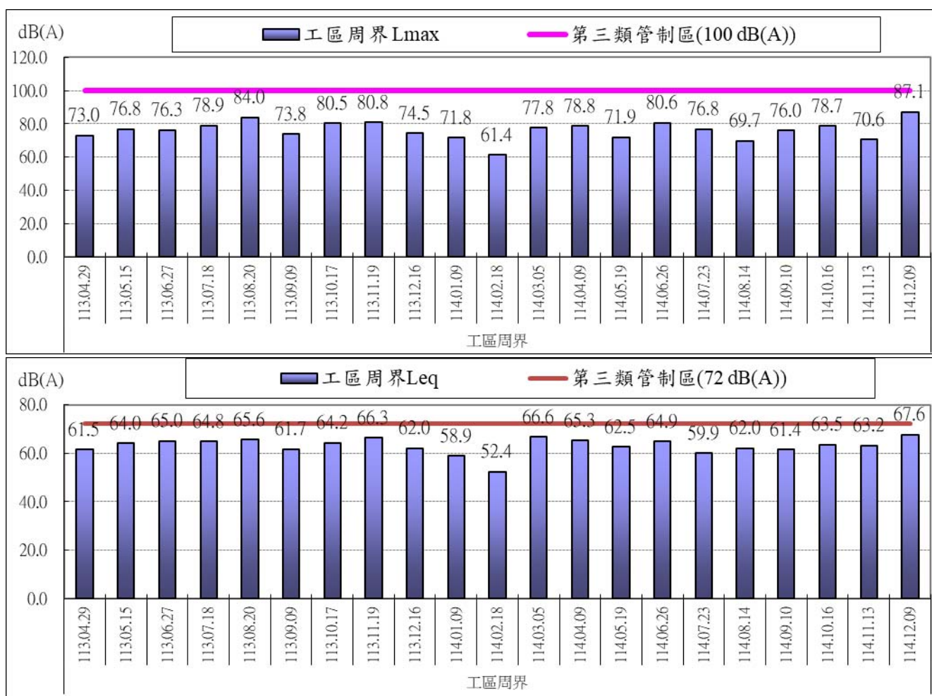
圖 2.10-1 營建噪音 L max 及 L eq 監測成果圖
