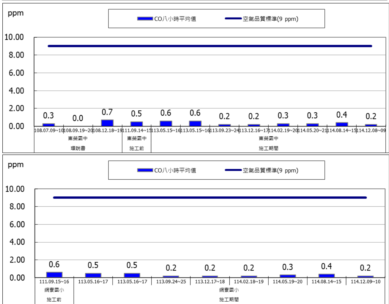
圖 2.1-11 一氧化碳(CO)測值 8 小時平均值監測成果圖
