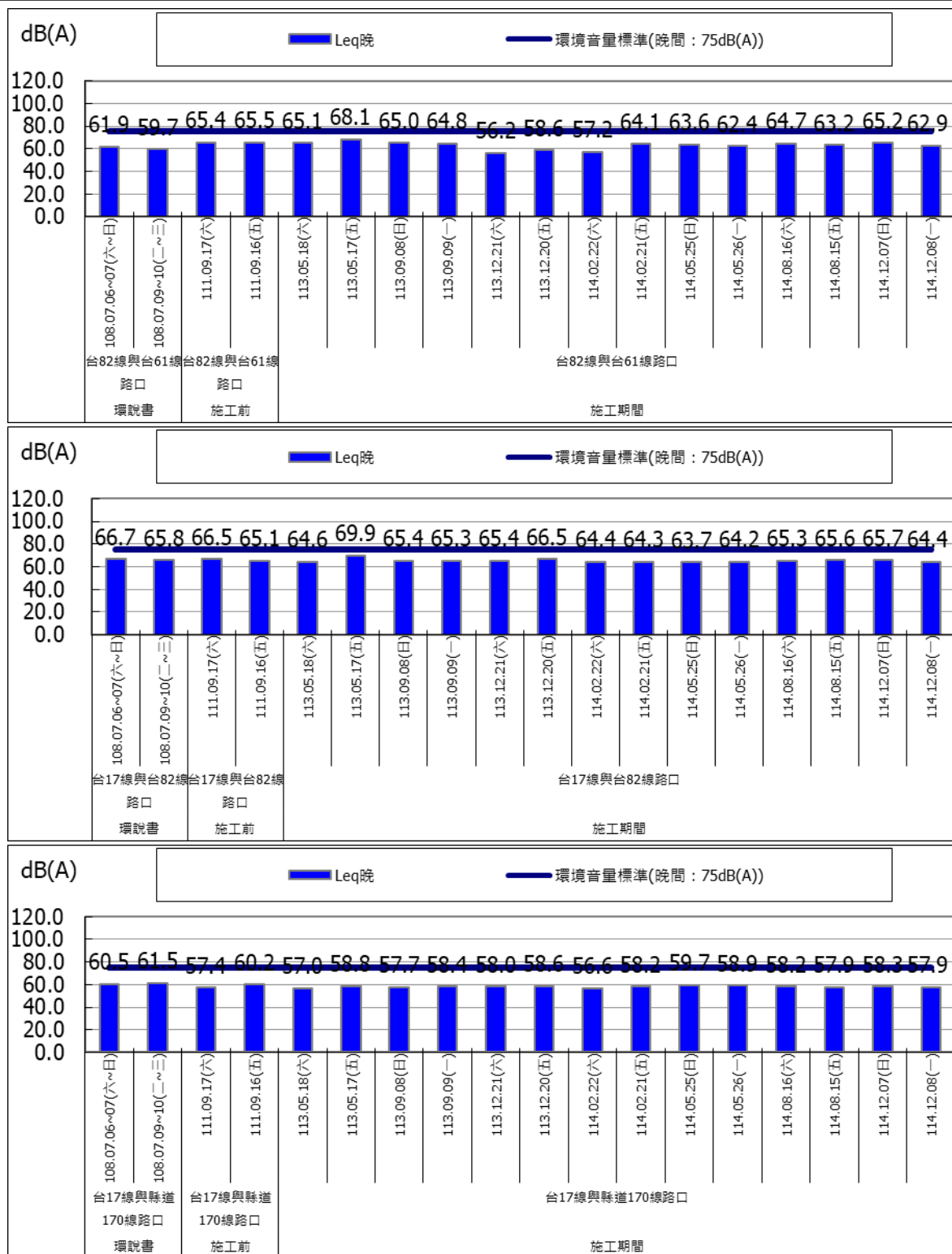
圖 2.2-2 各測站( L_{eq} 晚)環境噪音監測成果圖
