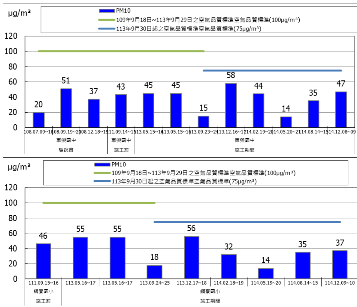
圖 2.1-1 懸浮微粒(PM 10 )測值日平均值監測成果圖
