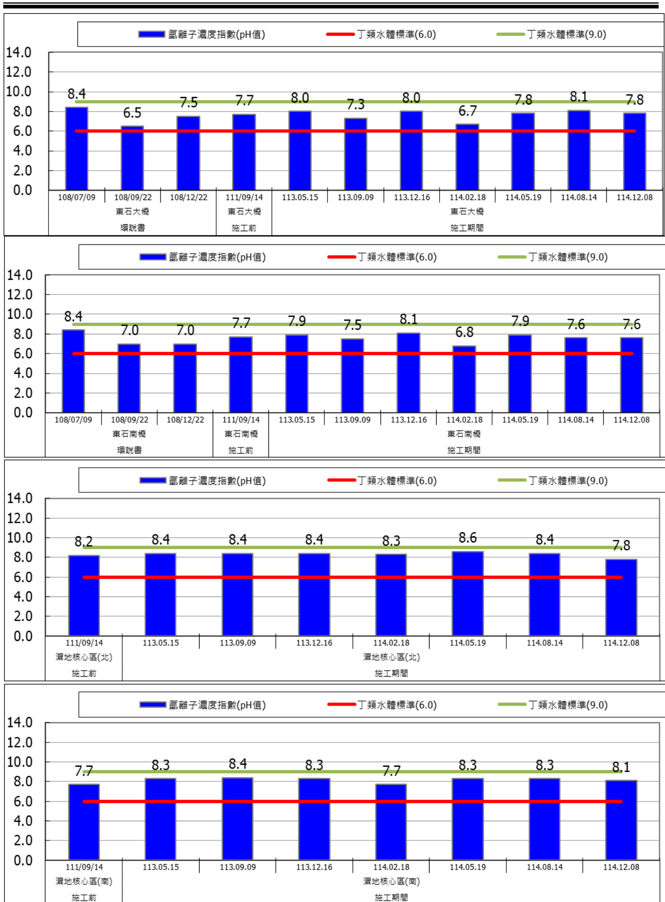
圖 2.3-2 地表水監測成果圖(pH 指數)
