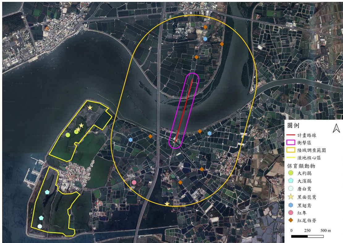
圖 2.8-3 保育類動物分布圖(113 年 10 月 施工期間)
