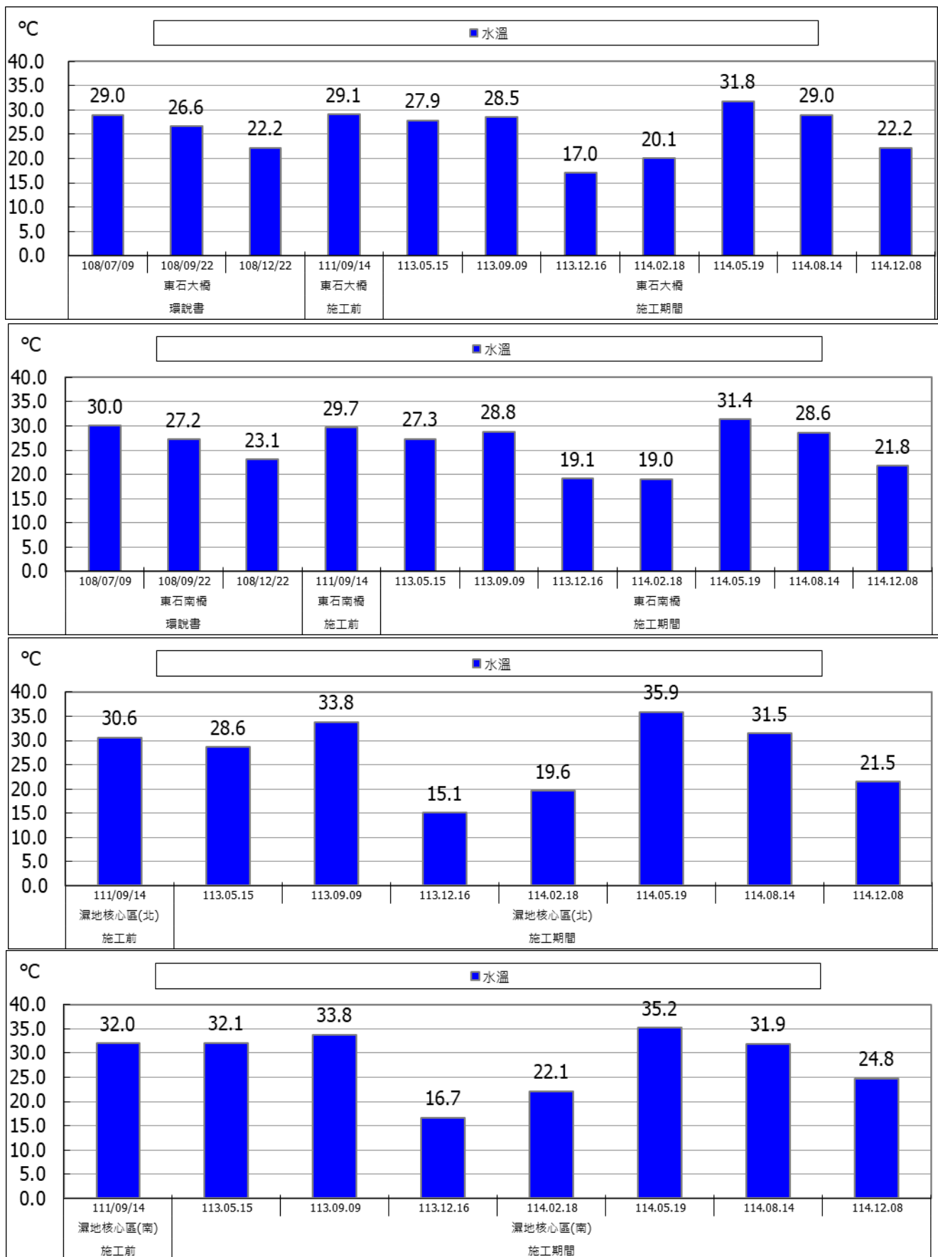
圖 2.3-1 地表水監測成果圖(水溫)
