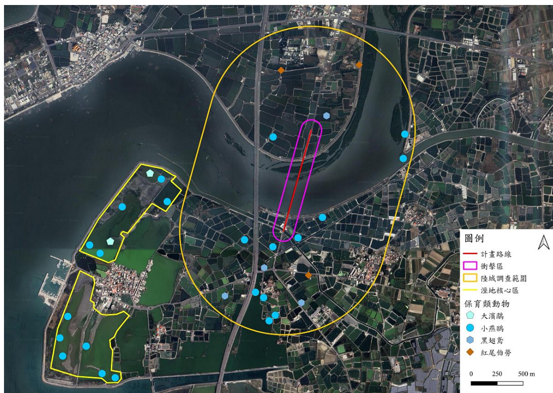
圖 2.8-3 保育類動物分布圖(114 年 4 月 施工期間)
