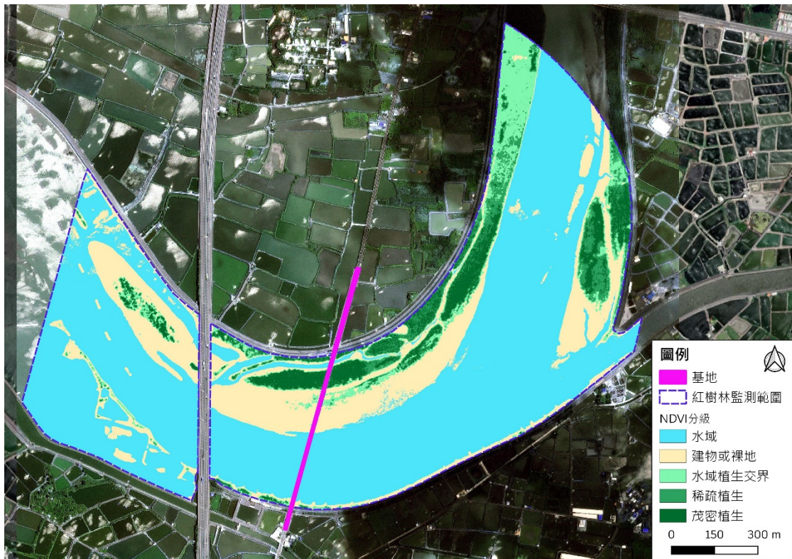
圖 2.5-3.1 紅樹林監測範圍與 NDVI 數值分級圖(施工前 111 年 8 月)
