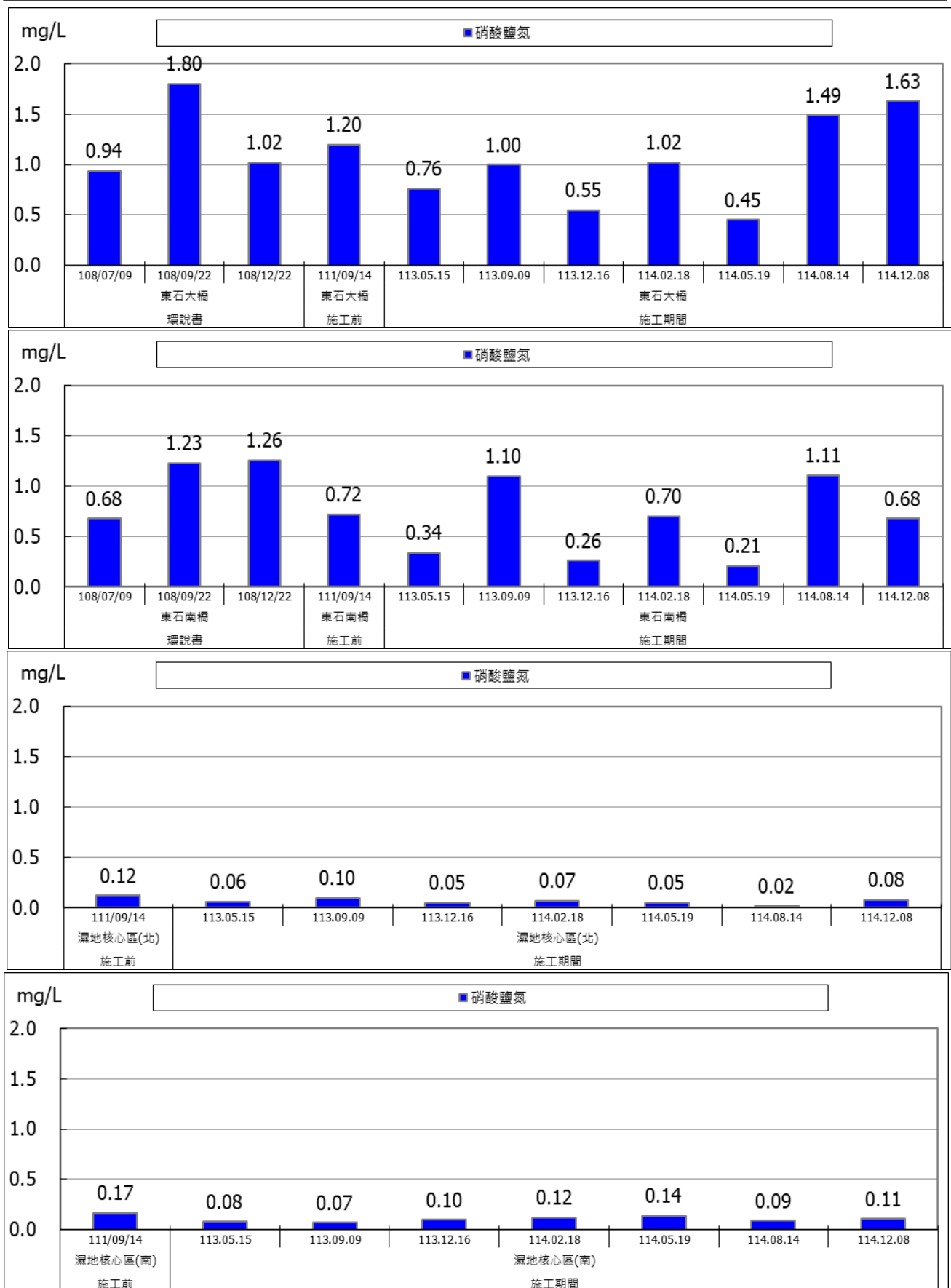
圖 2.3-7 地表水監測成果圖(硝酸鹽氮)
