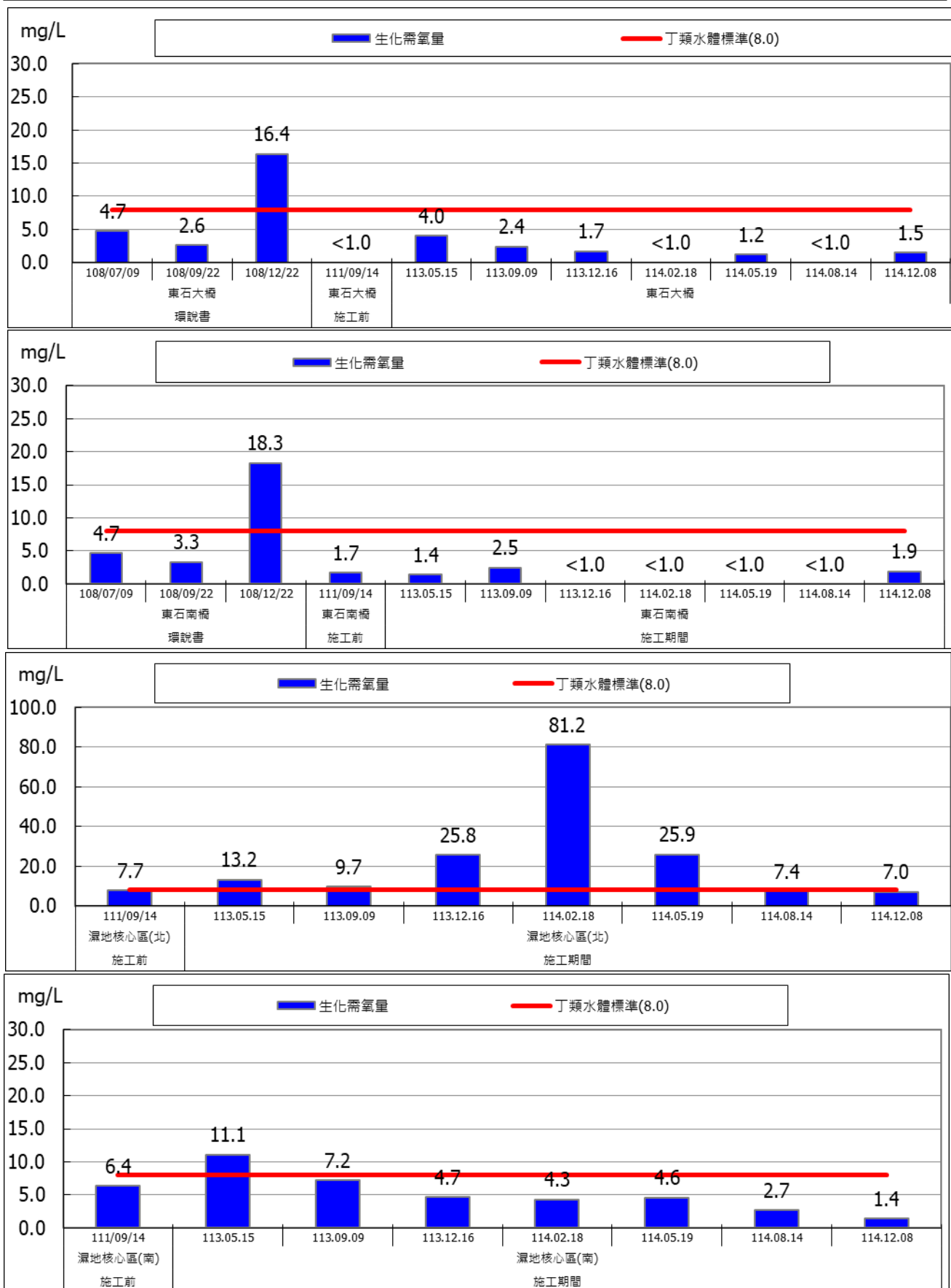
圖 2.3-4 地表水監測成果圖(生化需氧量)
