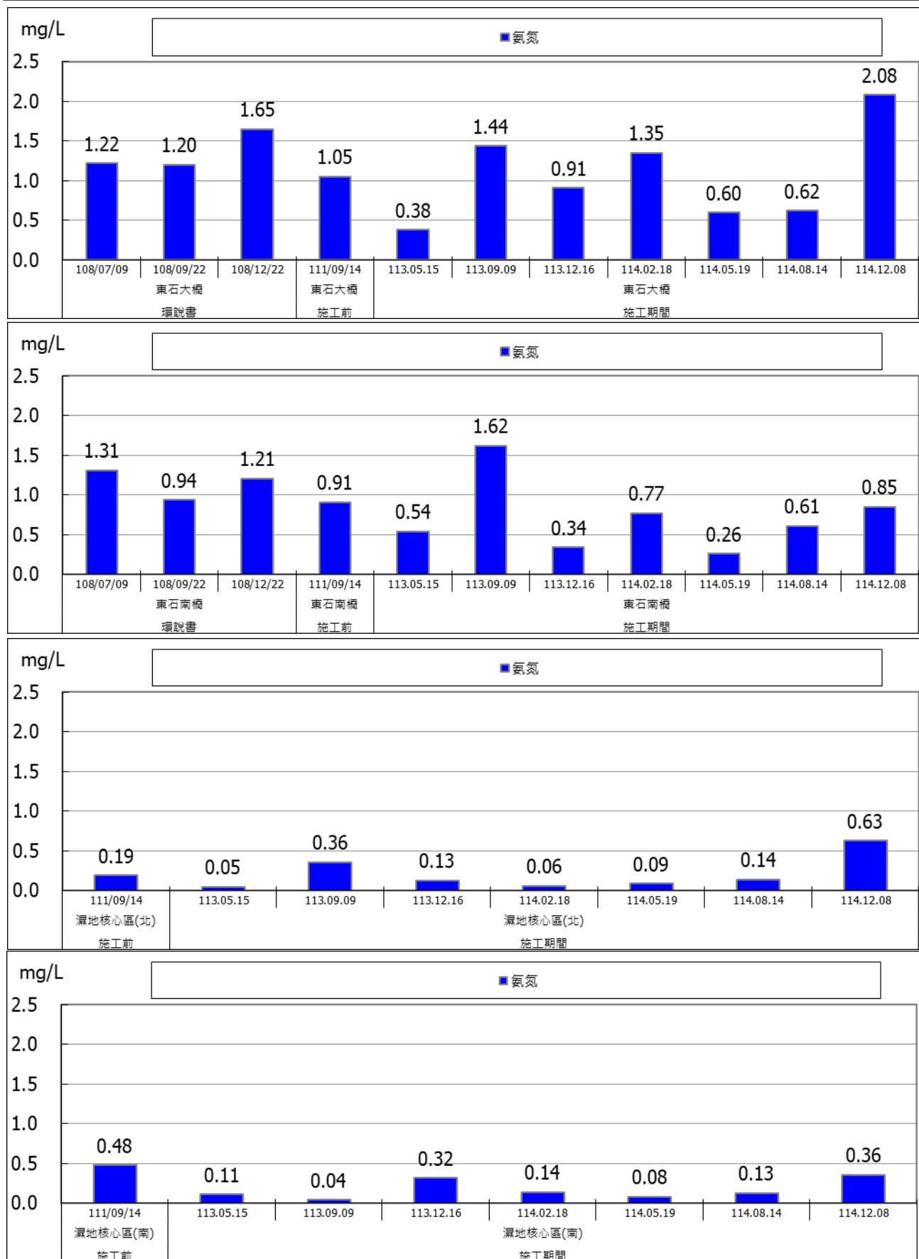
圖 2.3-8 地表水監測成果圖(氨氮)
