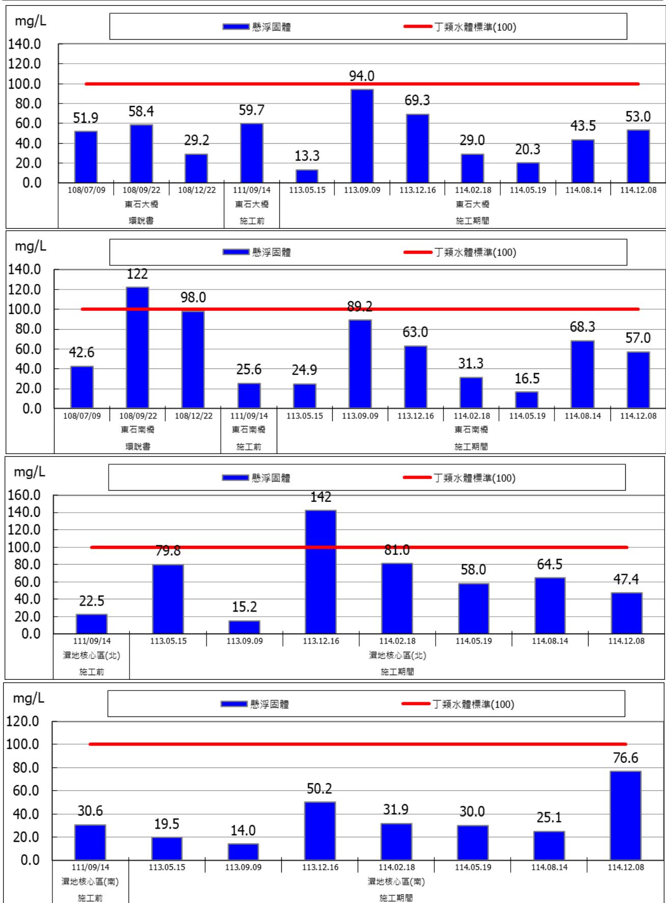
圖 2.3-6 地表水監測成果圖(懸浮固體)
