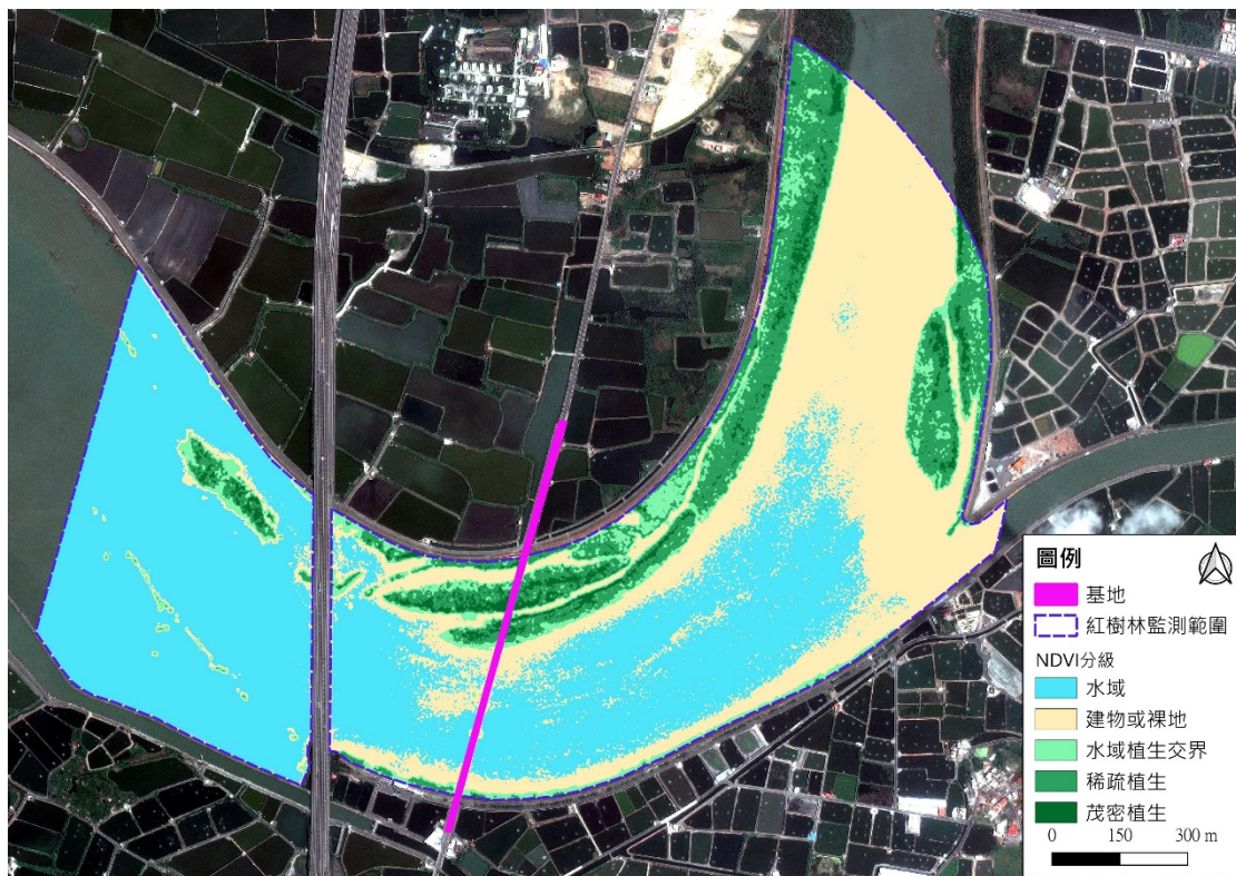
圖 2.5-3.3 紅樹林監測範圍與 NDVI 數值分級圖(施工期間 114 年 8 月)
