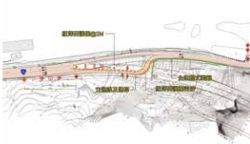
● 仁水隧道北洞口第三階段交通維持設施平面圖
