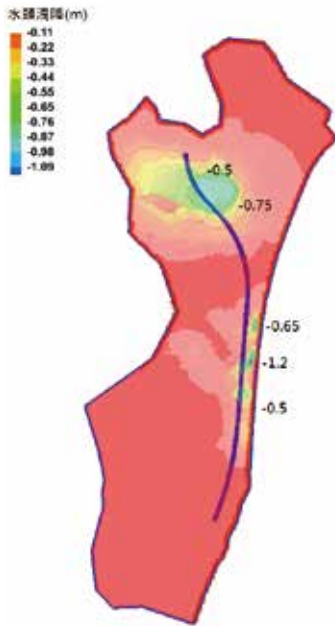
觀音隧道前階段(102年12月) 之地下水總水頭洩降分布情形 (單位:公尺)
