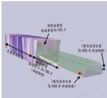
● 7K+785.4 TSP震波探測 -三維成果示意圖
