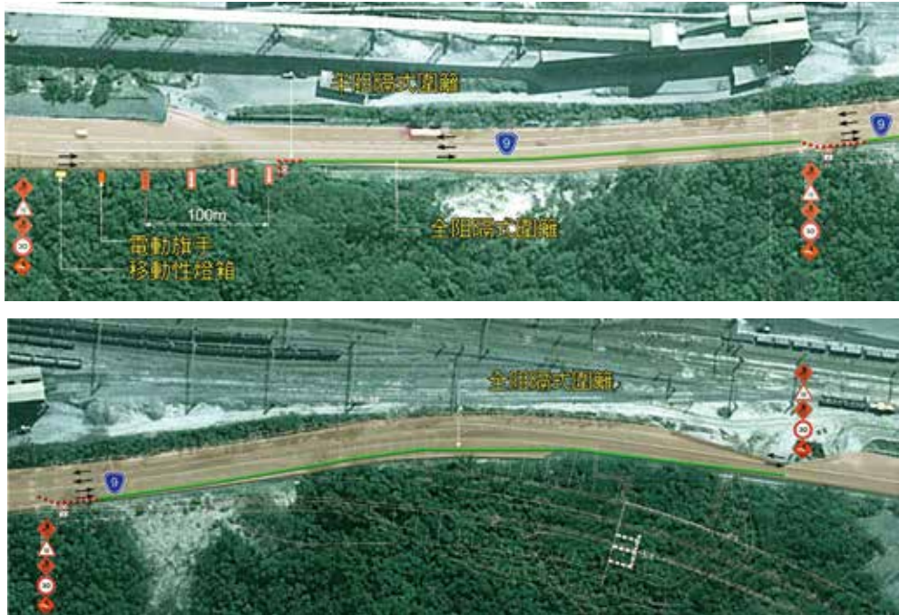
● 仁水隧道北洞口第一階段交通維持設施平面圖
