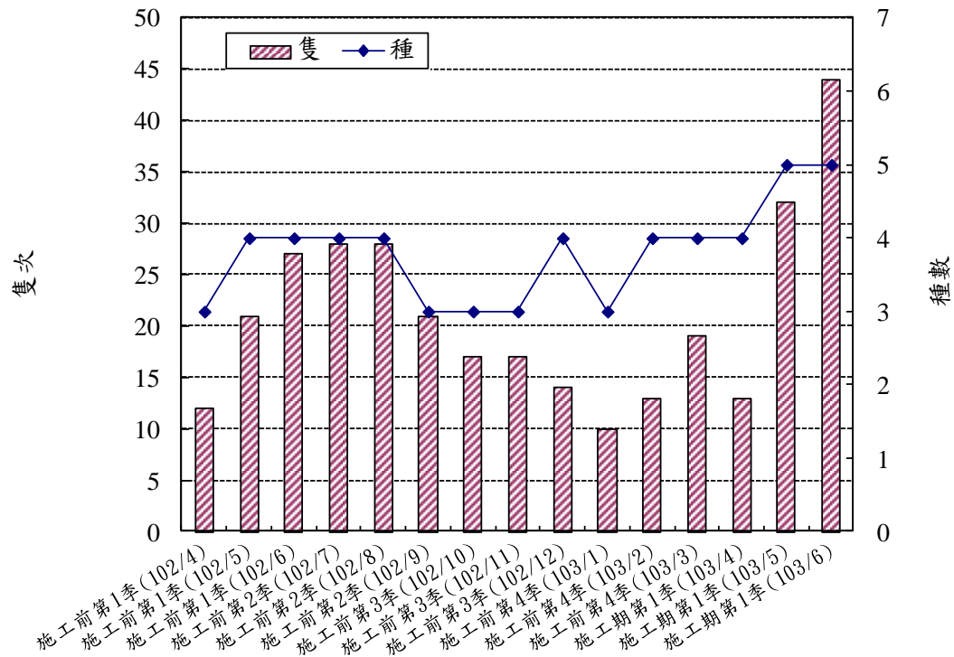
圖 3-1.4、兩棲類調查歷次比較圖
