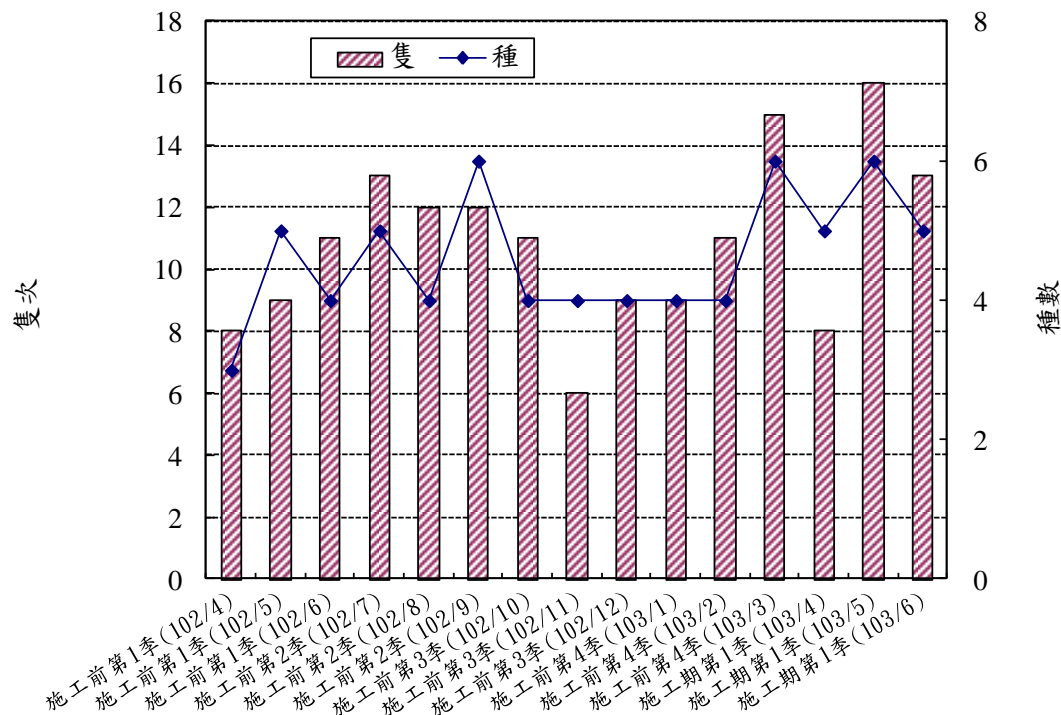
圖 3-1.5、爬蟲類調查歷次比較圖
