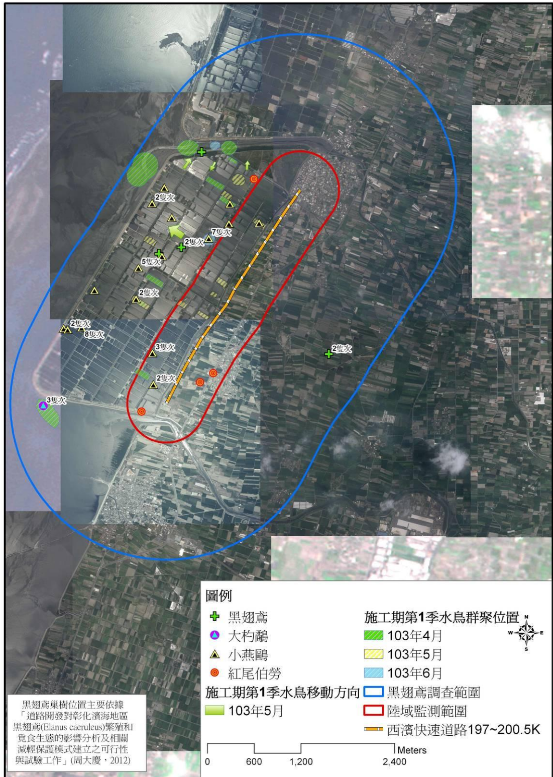
圖 2-1.1、施工期第 1 季保育類動物與水鳥群聚發現位置(103 年 4~6 月)
