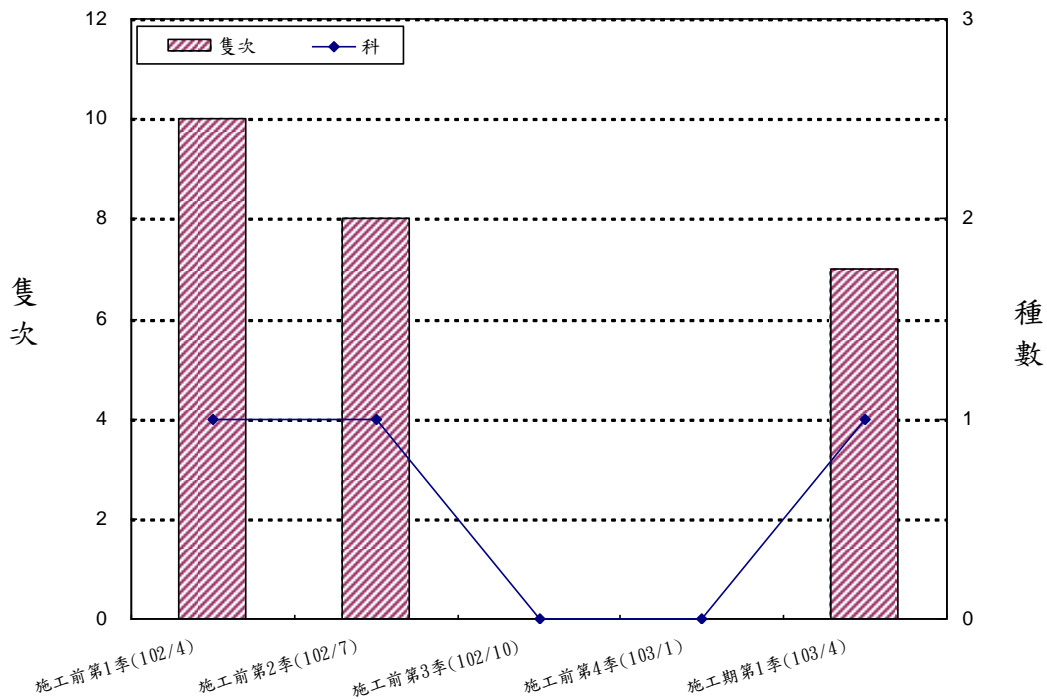
圖 3-1.9、水域生物水生昆蟲調查歷年各季比較圖
