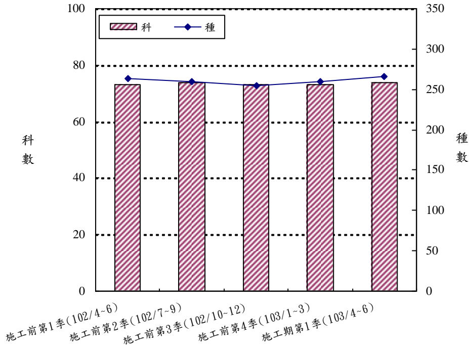
圖 3-1.1、陸域植物調查歷年各季比較圖
