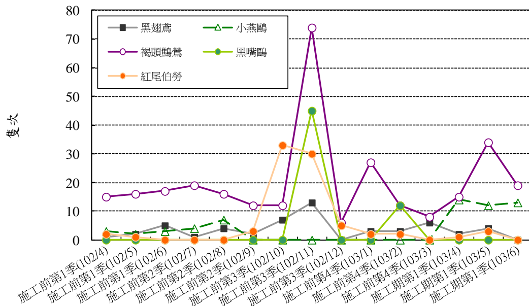
圖 3-1.6.1、指標物種歷次比較圖
