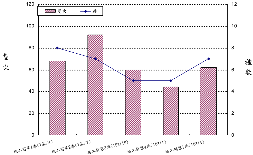
圖 3-1.8、水域生物蝦蟹螺貝類調查歷年各季比較圖
