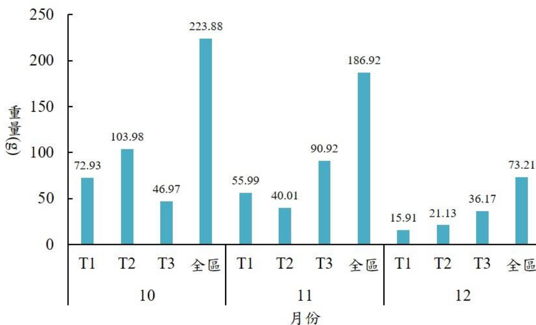
圖 2.1-2 落葉量總重量本季各月份變化圖
