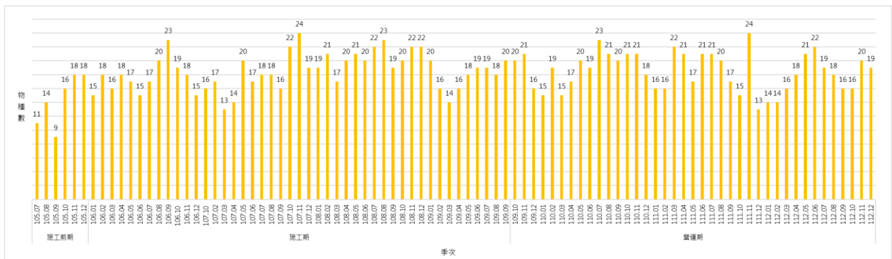
圖 2.2-3 底棲動物歷次物種數變化圖
