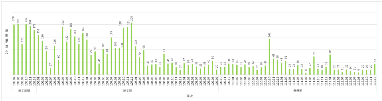
圖 2.2-2 鷺鷥歷次數量變化圖
