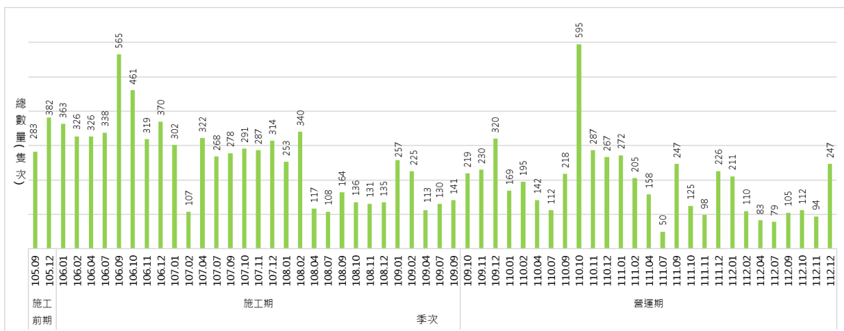
圖 2.3-2 候鳥歷次數量變化圖
