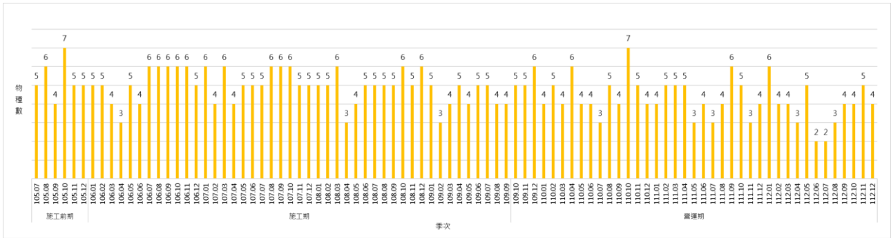
圖 2.2-1 鷺鷥歷次物種數變化圖
