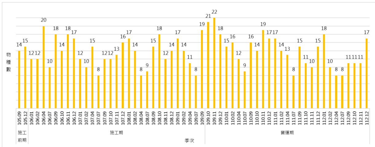
圖 2.3-1 候鳥歷次物種數變化圖
