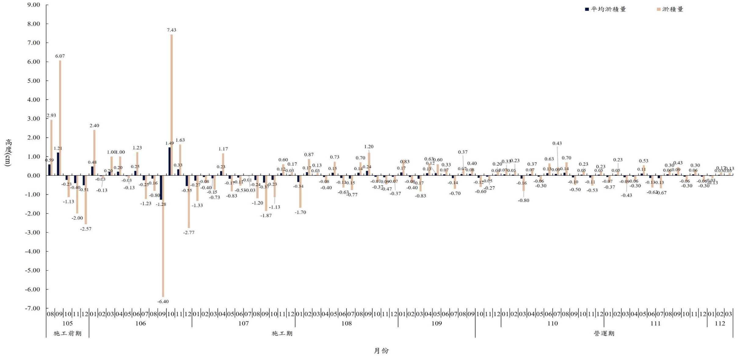
圖 2.1-6 淤泥高度各月份變化圖
