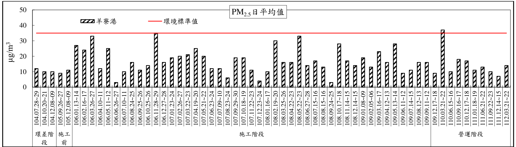
圖 2.4-1 羊寮港空氣品質監測成果趨勢圖
