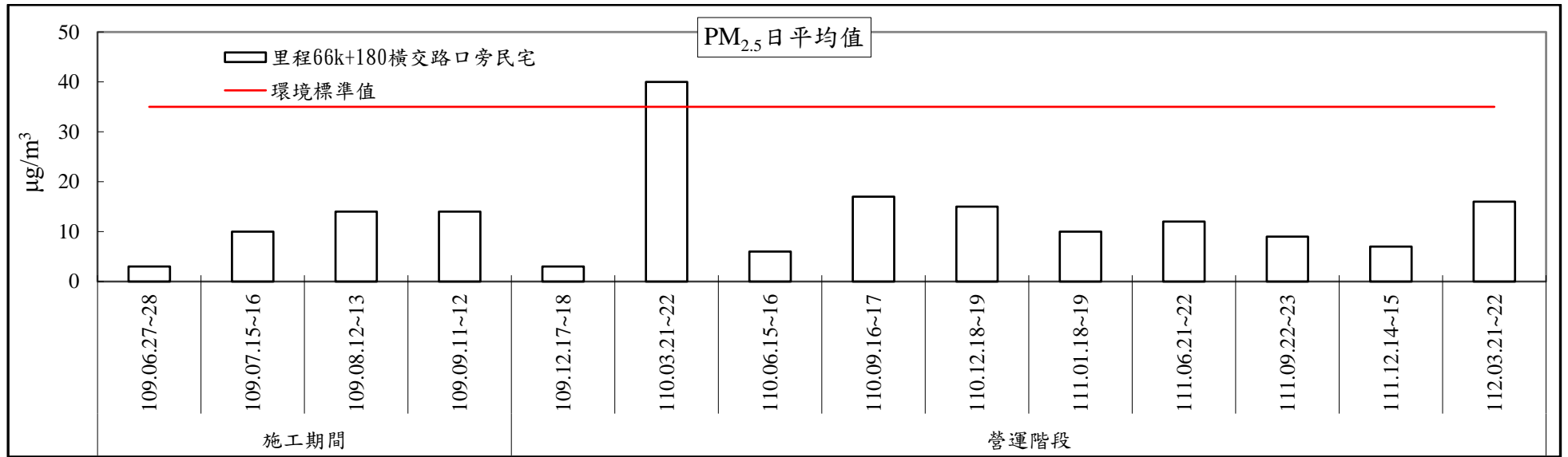
圖 2.4-2 里程 66k+180 橫交路口旁民宅空氣品質監測成果趨勢圖
