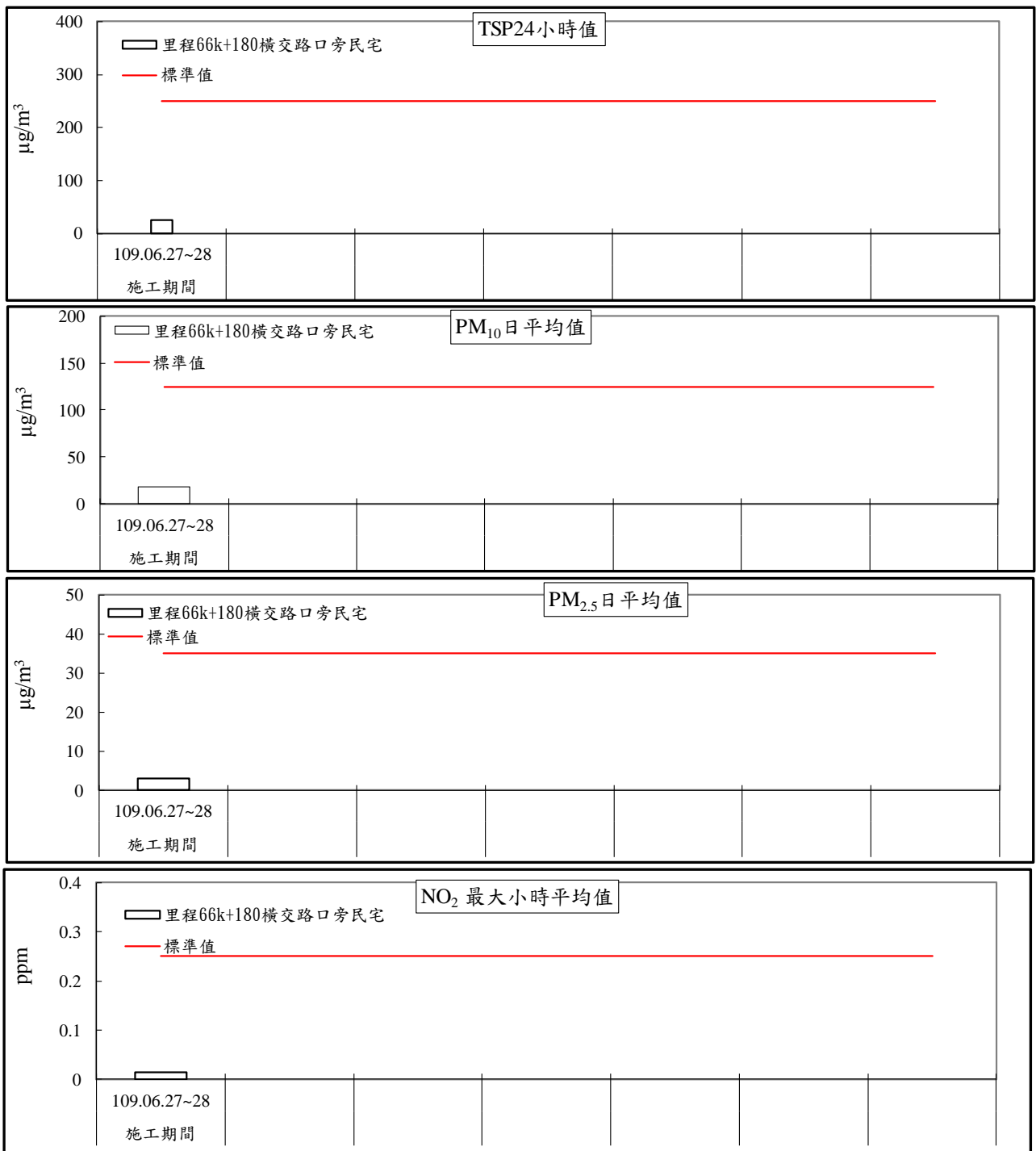
圖 2.8-2 里程 66k+180 橫交路口旁民宅空氣品質監測成果趨勢圖(1/2)
