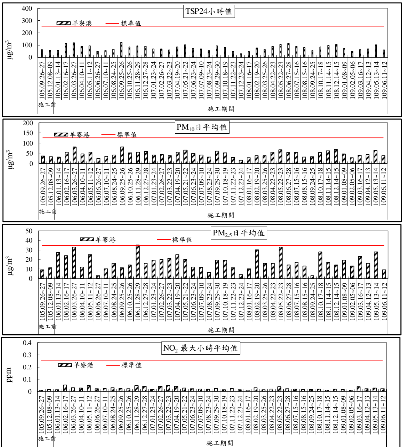
圖 2.8-1 羊寮港空氣品質監測成果趨勢圖(1/2)
