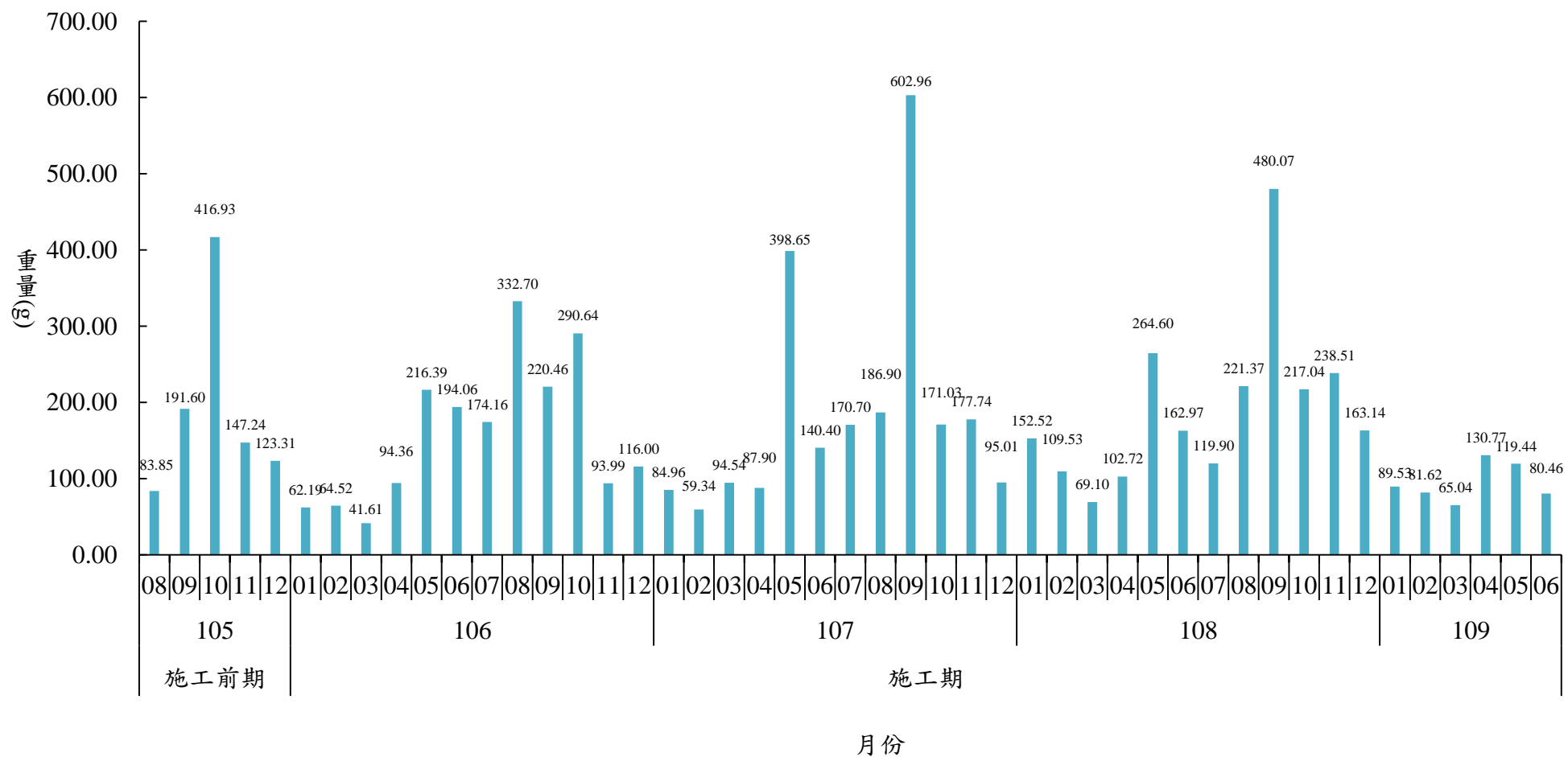
圖 2.5-5 落葉量總重量歷次各月份變化圖
