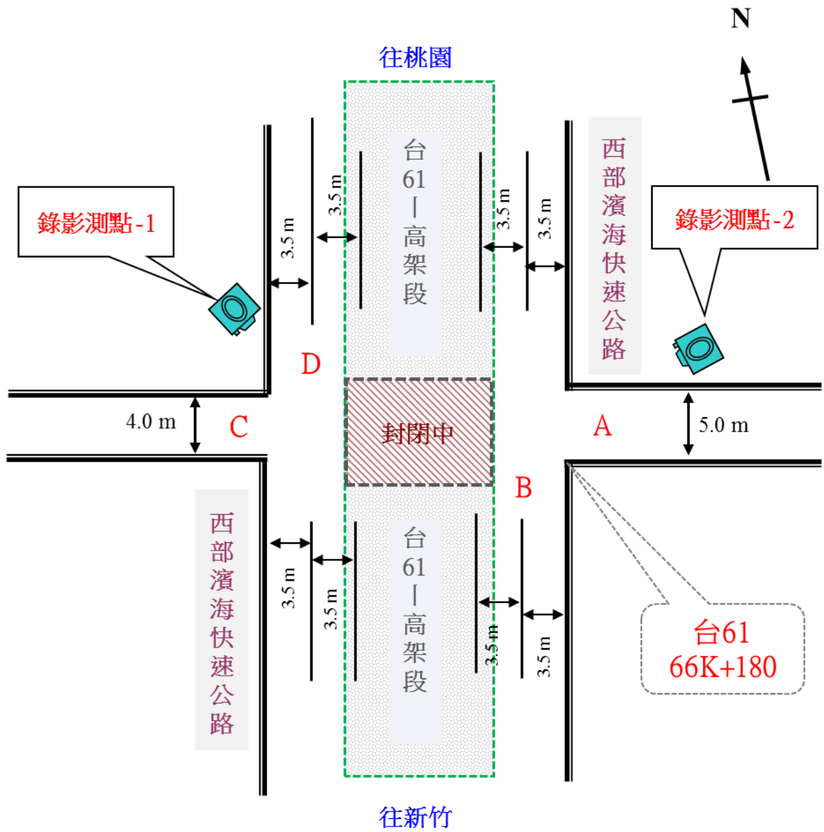
圖 2.11-1 交通流量量測點位置圖
