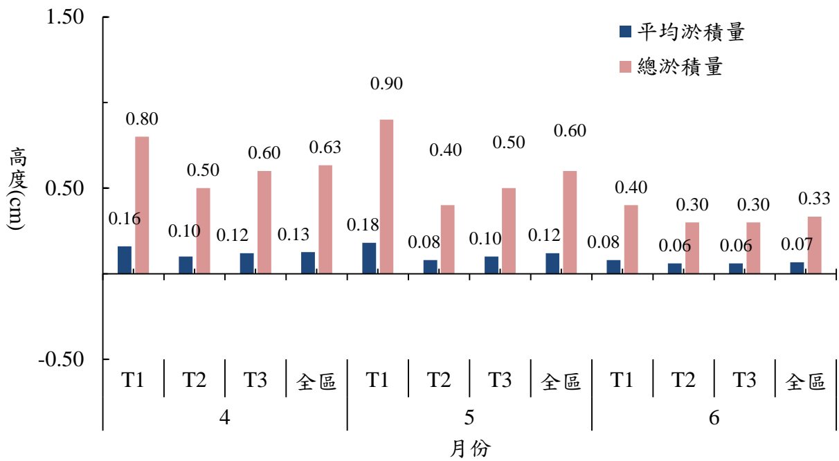
圖 2.5-3 淤泥高度本季各月份變化圖
