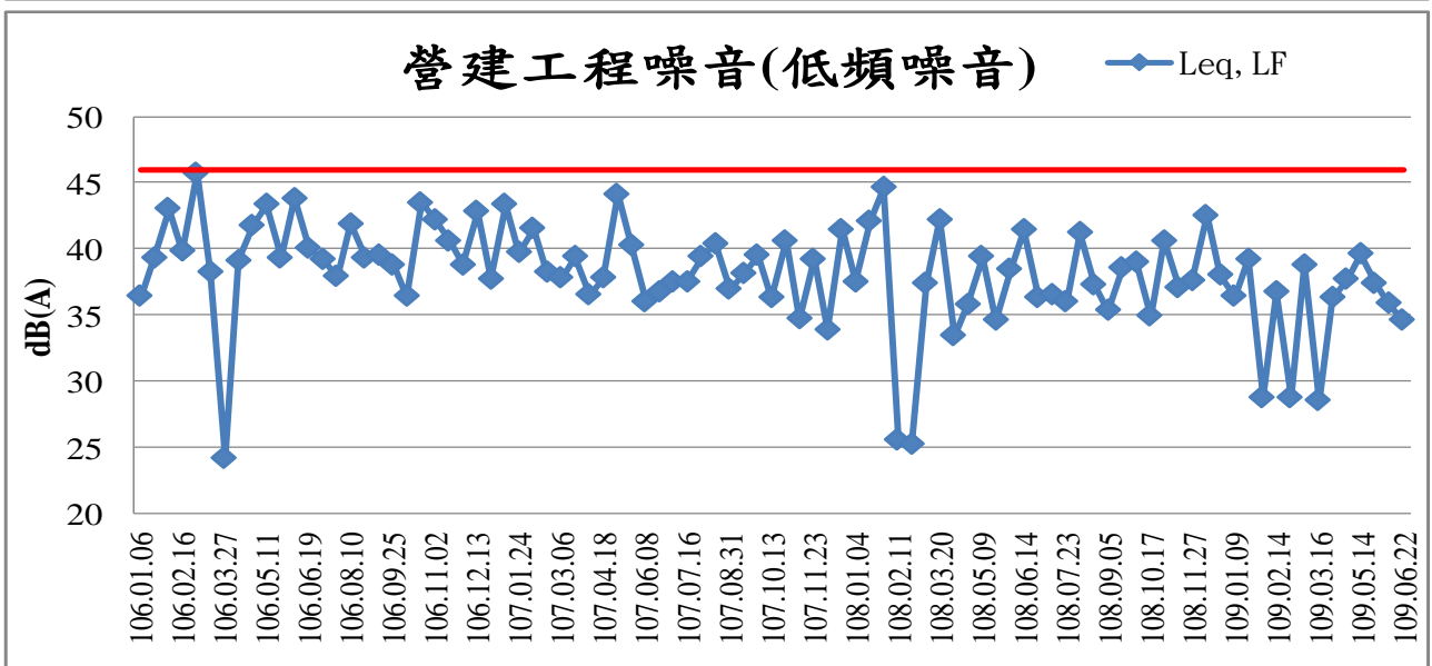
圖 2.3-1 營建工程噪音監測成果趨勢圖
