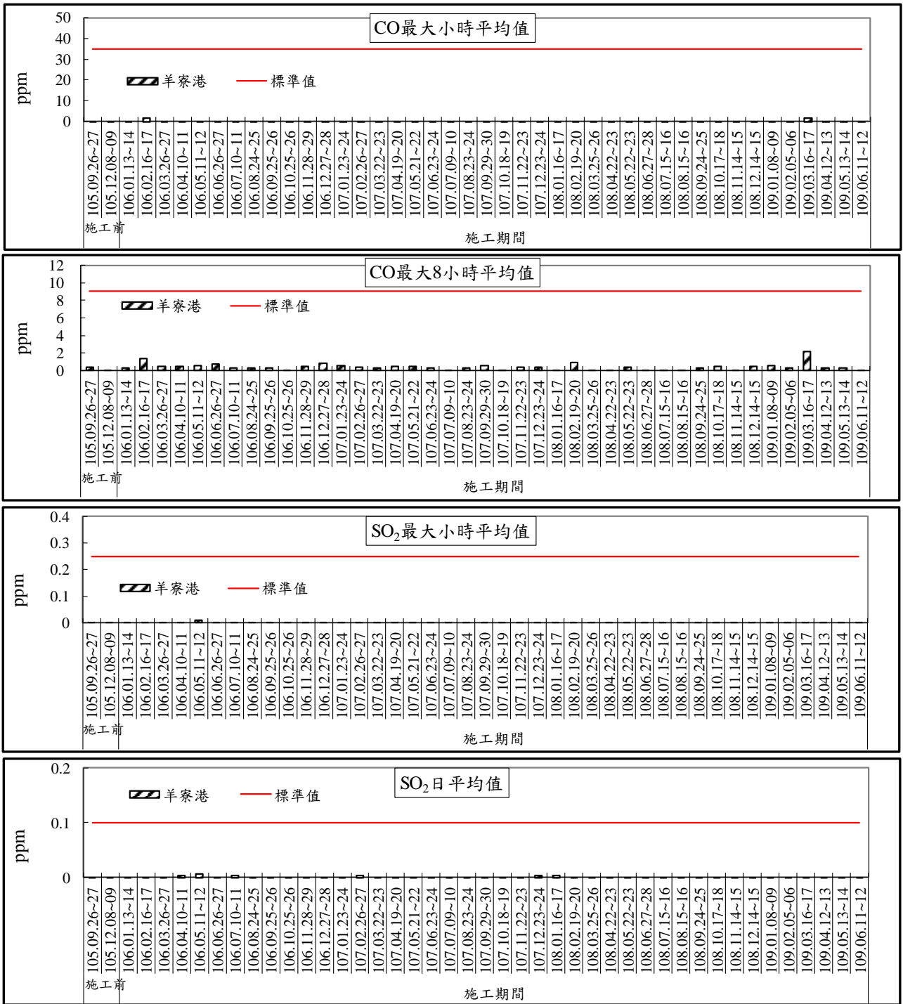
圖 2.8-1 羊寮港空氣品質監測成果趨勢圖(2/2)
