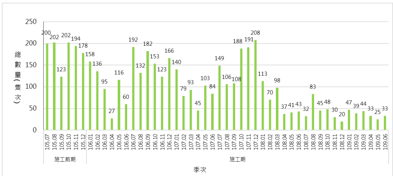
圖 2.6-2 鷺鷥歷次數量變化圖
