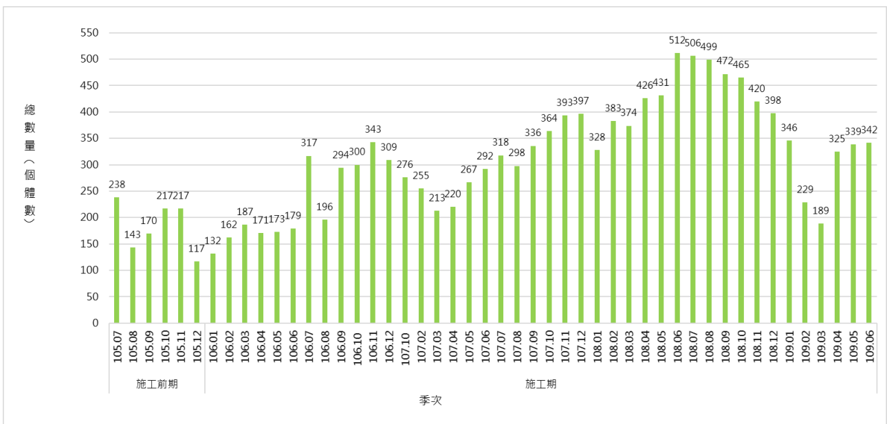
圖 2.6-4 底棲動物歷次數量變化圖
