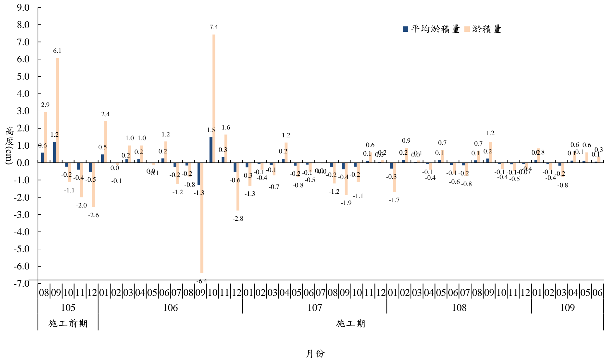
圖 2.5-6 淤泥高度各月份變化圖
