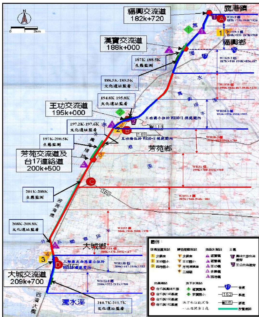
註：本計畫路線環境監測依上圖粗線範圍計分為5標，①182K+720-90K+024.487②190K+024.487-195K+995③195K+995-202K-940④202K+940-209K+17⑤209K-117-212K-700。交通量調查計分為2標，①台17線與員林大排及152線路口②台17線與148線及150線路口。生態監測計分為3標，①187K-188.5K②197K-200.5K③201K-208K。文化遺址監看分為5處①188.5K-189.5K②194.8K-195.8K③197.2K-197.6K④208K-208.8K⑤210.7K-211.7K。
