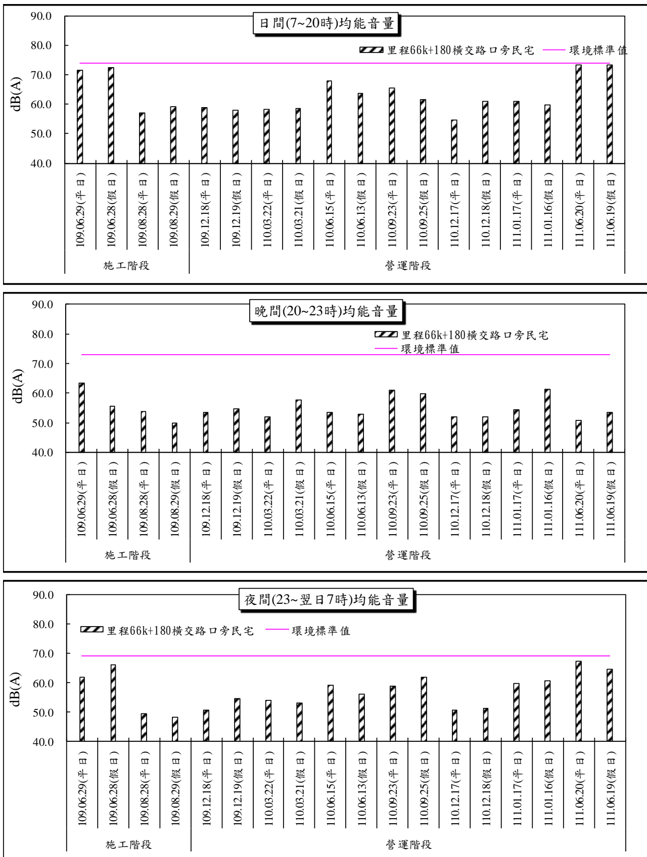
圖 2.9-3 里程 66k+180 橫交路口旁民宅測站噪音監測結果變化趨勢圖
