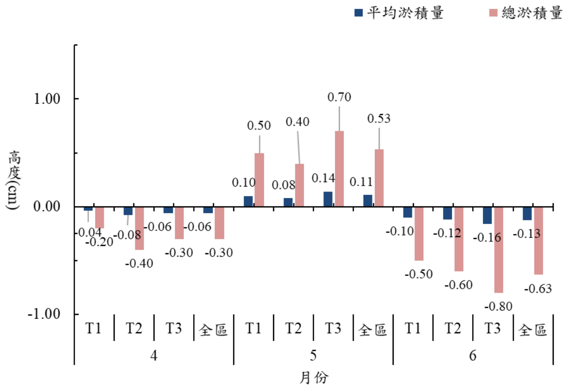
圖 2.5-3 淤泥高度本季各月份變化圖
