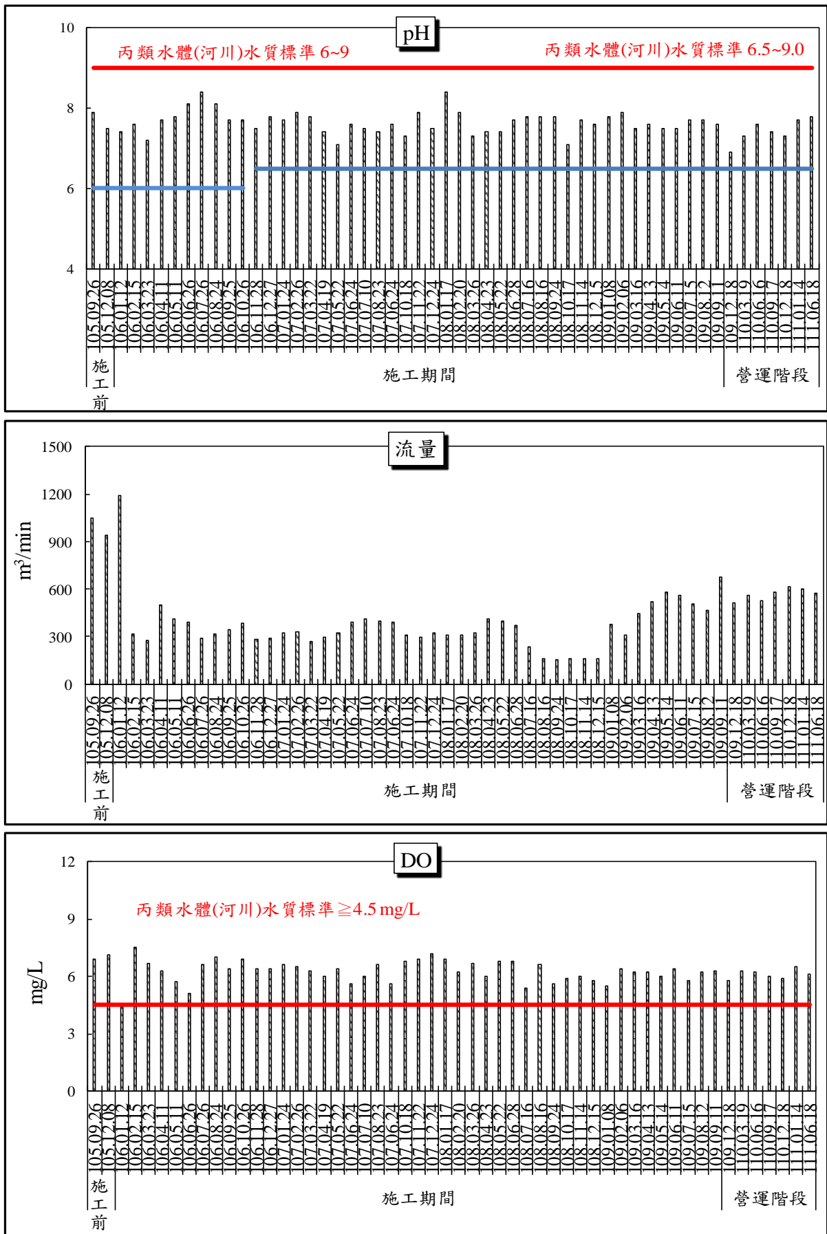
圖 2.10-1 新豐溪紅樹林橋監測結果變化趨勢圖(1/3)
