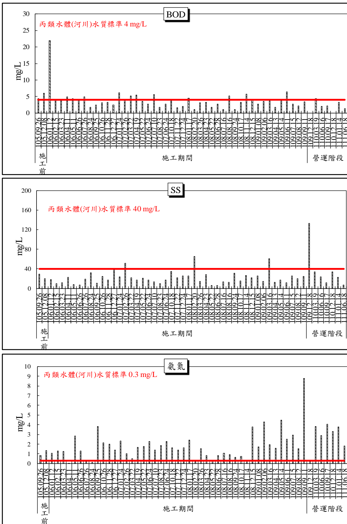
圖 2.10-1 新豐溪紅樹林橋監測結果變化趨勢圖(2/3)
