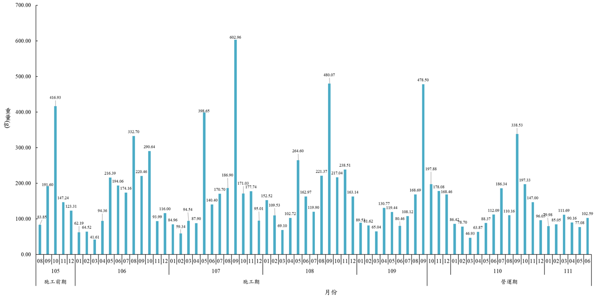
圖 2.5-5 落葉量總重量歷次各月份變化圖
