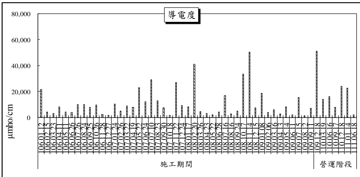
圖 2.10-2 池和橋監測結果變化趨勢圖(3/3)
