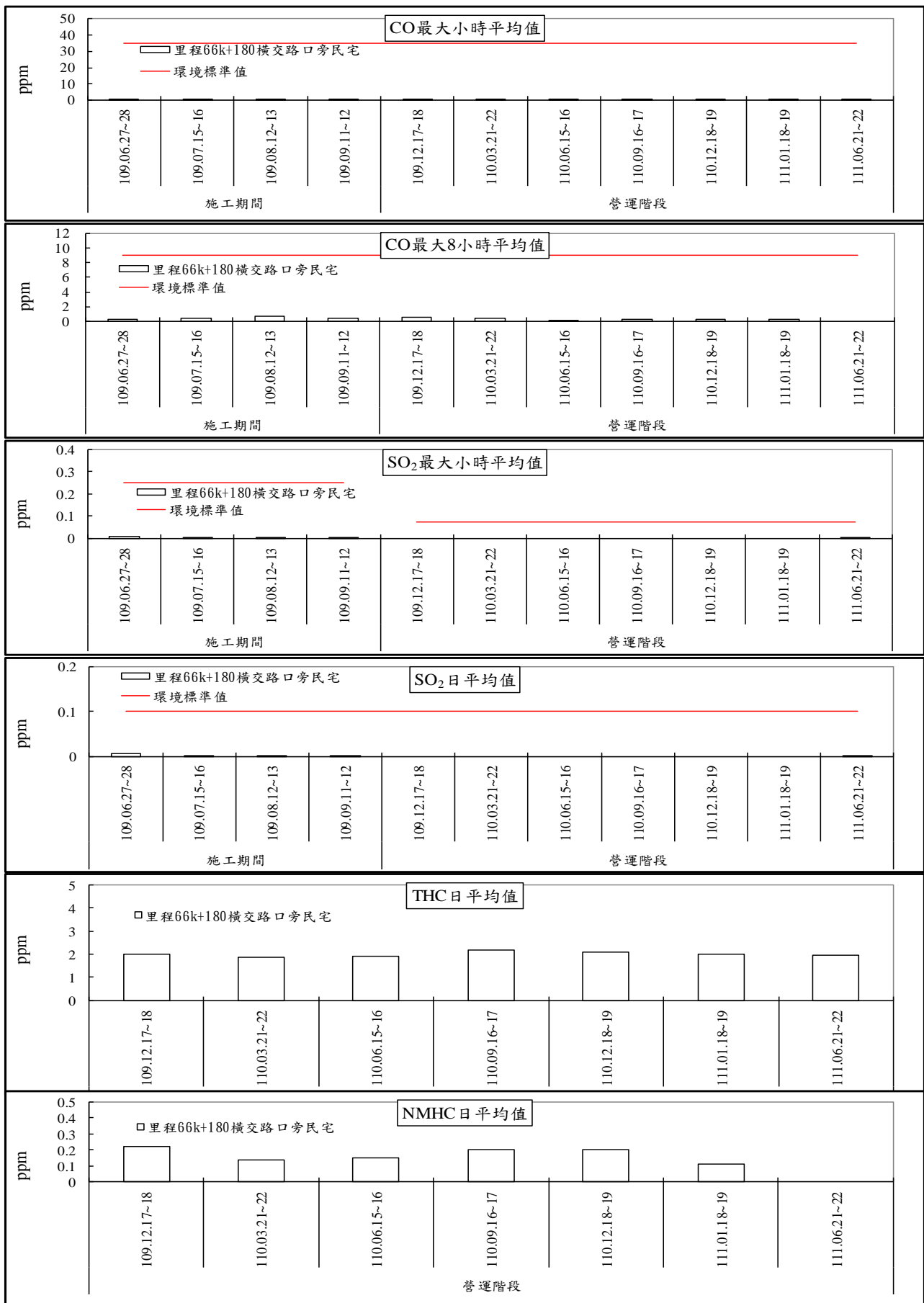
圖 2.8-2 里程 66k+180 橫交路口旁民宅空氣品質監測成果趨勢圖(2/2)
