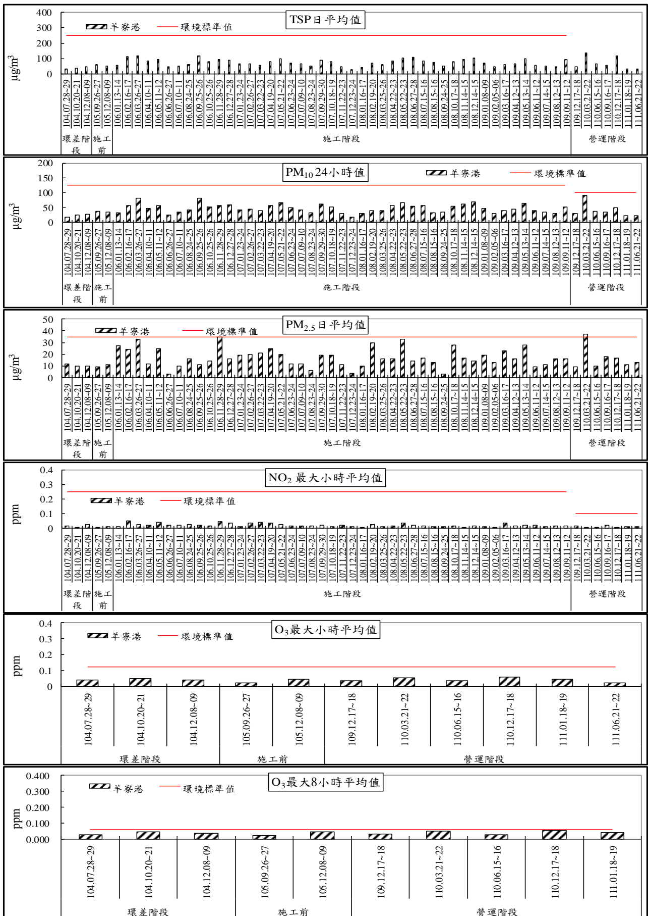
圖 2.8-1 羊寮港空氣品質監測成果趨勢圖(1/2)
