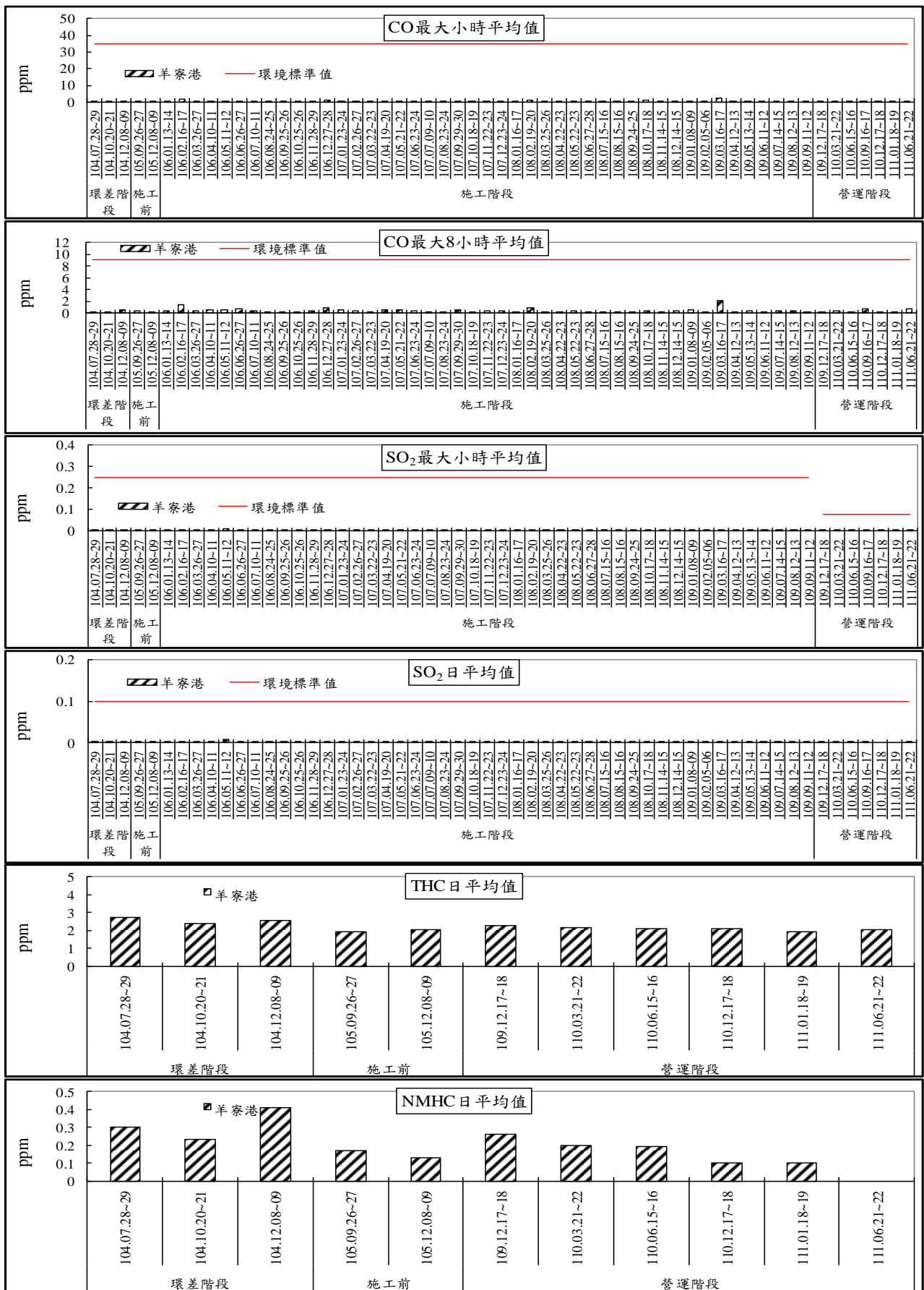
圖 2.8-1 羊寮港空氣品質監測成果趨勢圖(2/2)
