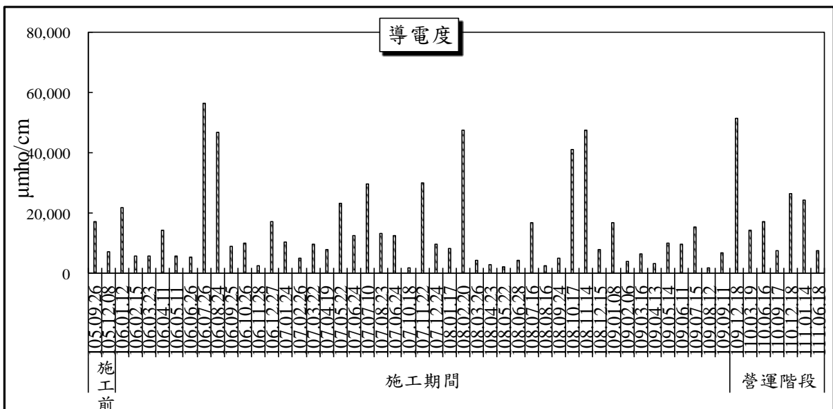
圖 2.10-1 新豐溪紅樹林橋監測結果變化趨勢圖(3/3)
