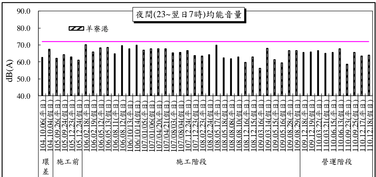
圖 2.9-1 羊寮港測站噪音監測結果變化趨勢圖
