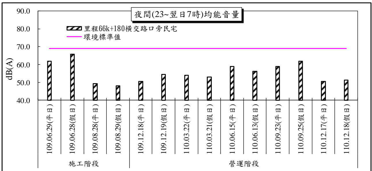
圖 2.9-3 里程 66k+180 橫交路口旁民宅測站噪音監測結果變化趨勢圖
