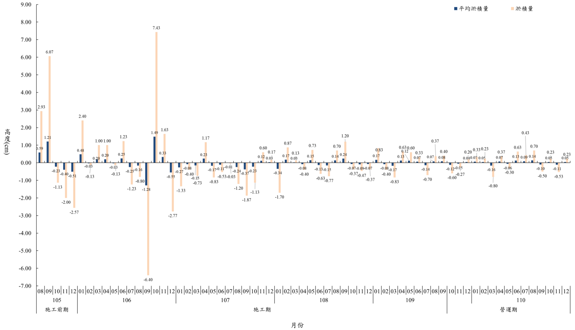
圖 2.5-6 淤泥高度各月份變化圖
