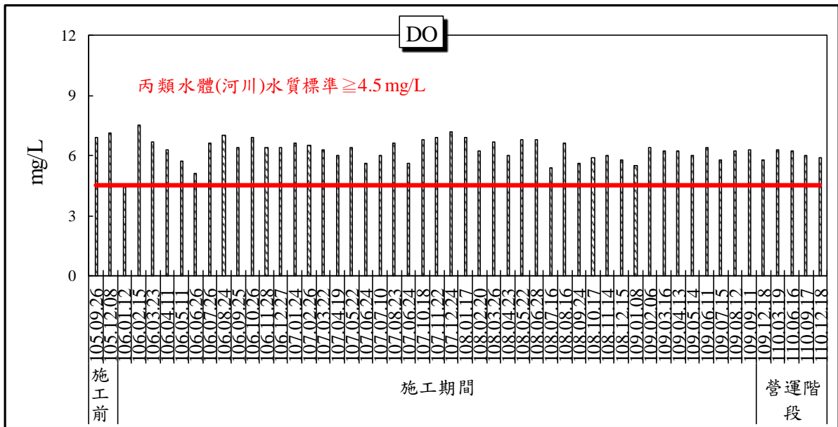
圖 2.10-1 新豐溪紅樹林橋監測結果變化趨勢圖(1/3)
