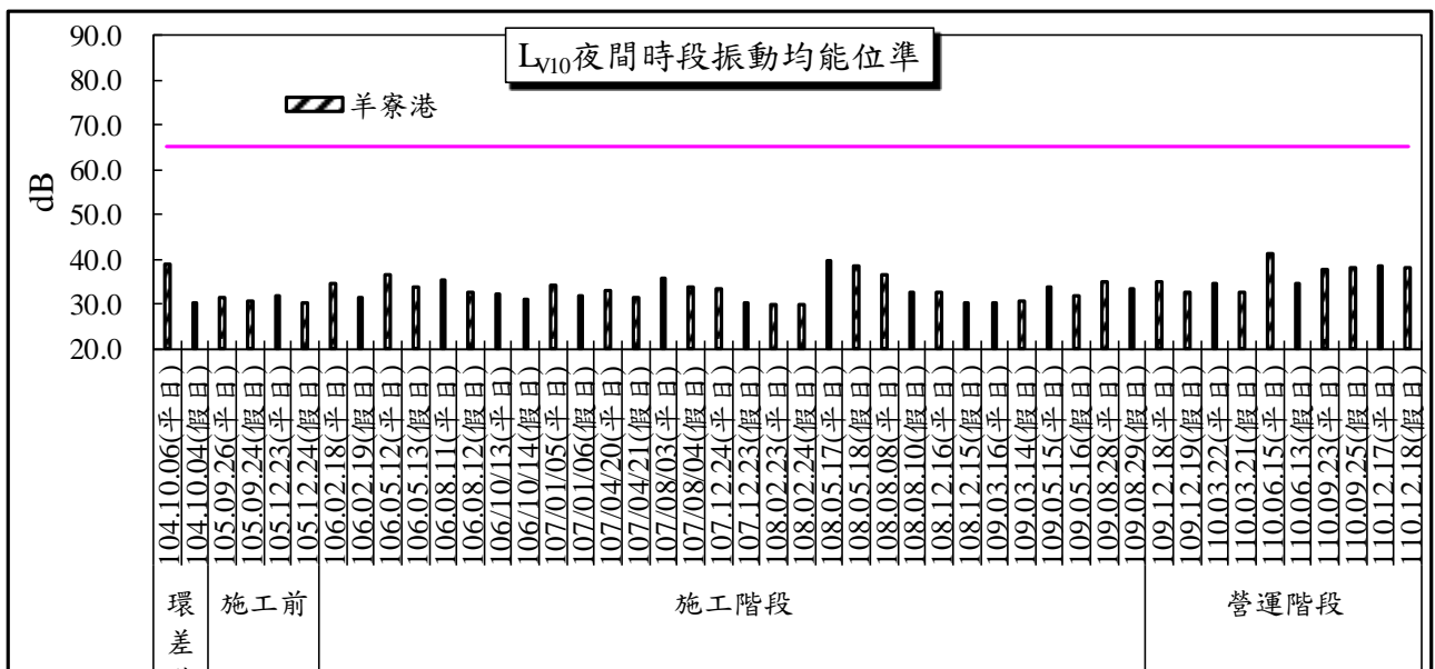
圖 2.9-2 羊寮港測站振動監測結果變化趨勢圖
