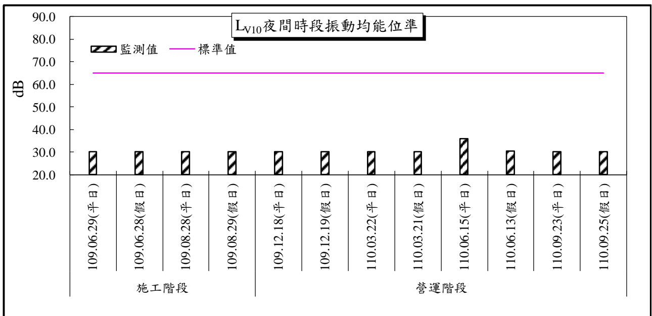
圖 2.9-4 里程 66k+180 橫交路口旁民宅測站振動監測結果變化趨勢圖
