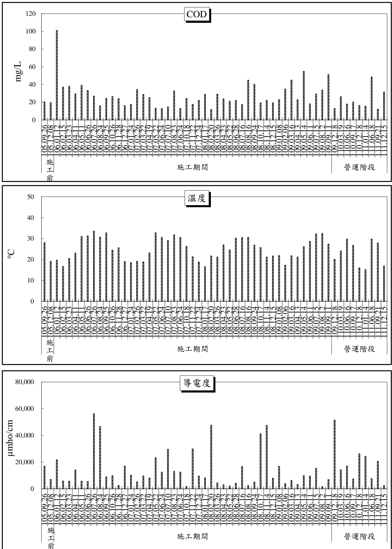
圖 2.10-1 新豐溪紅樹林橋監測結果變化趨勢圖(3/3)
