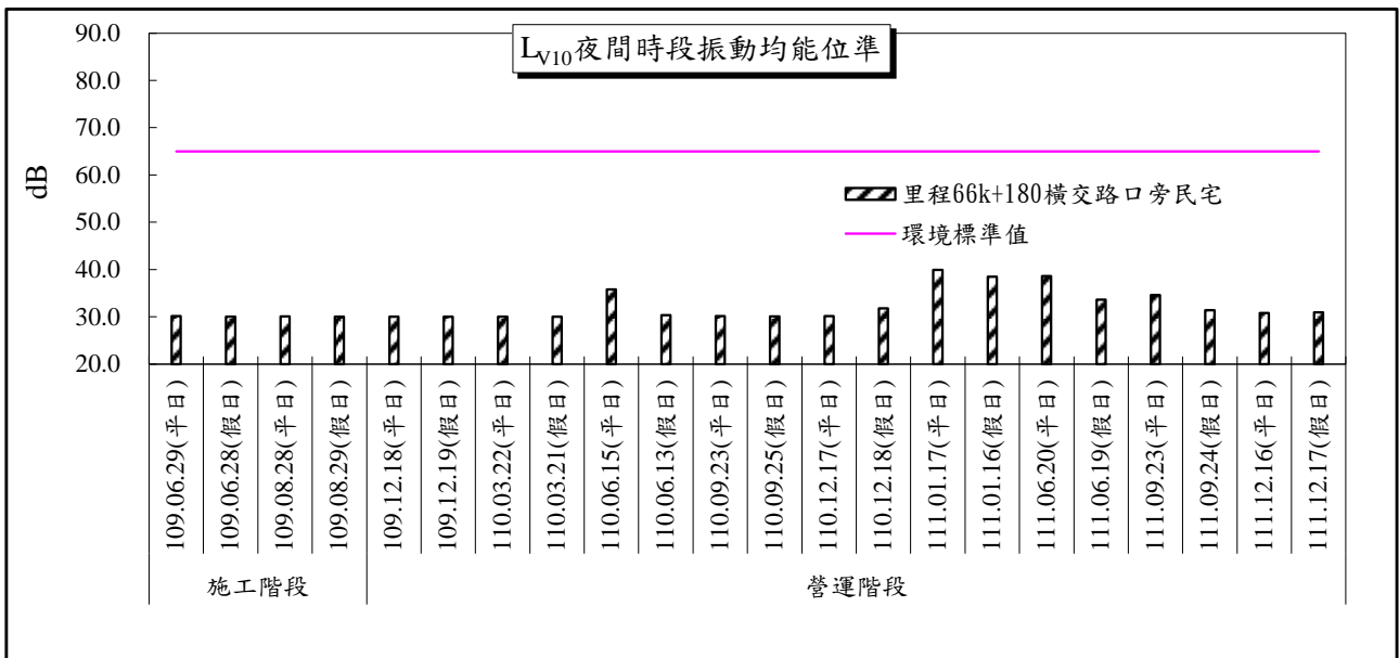
圖 2.9-4 里程 66k+180 橫交路口旁民宅測站振動監測結果變化趨勢圖
