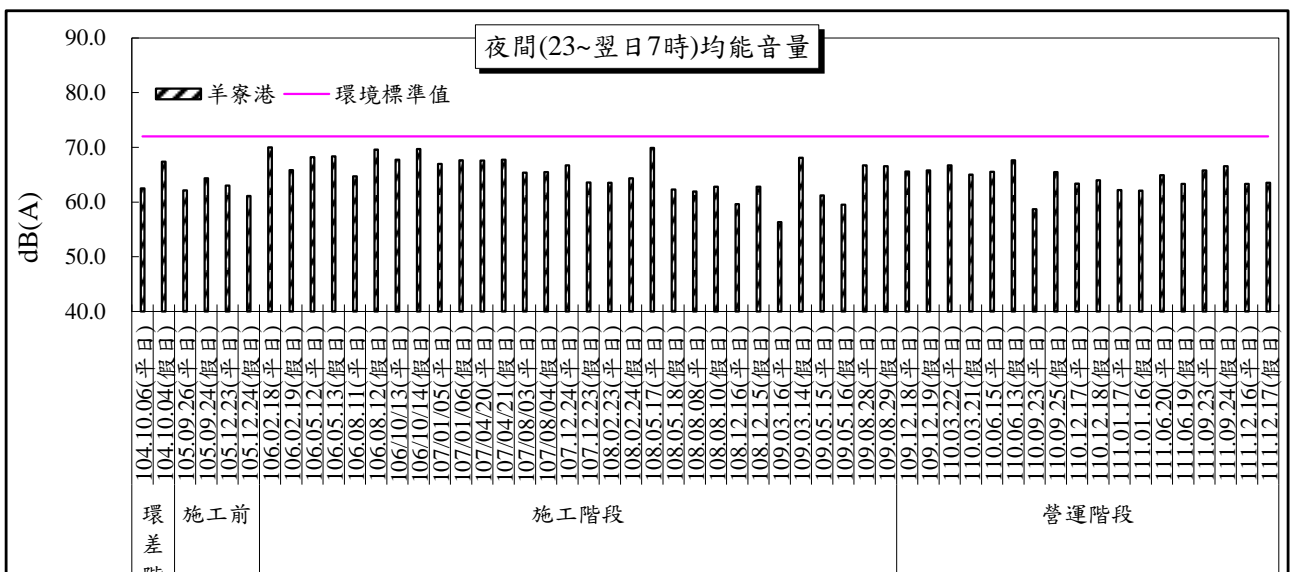
圖 2.9-1 羊寮港測站噪音監測結果變化趨勢圖
