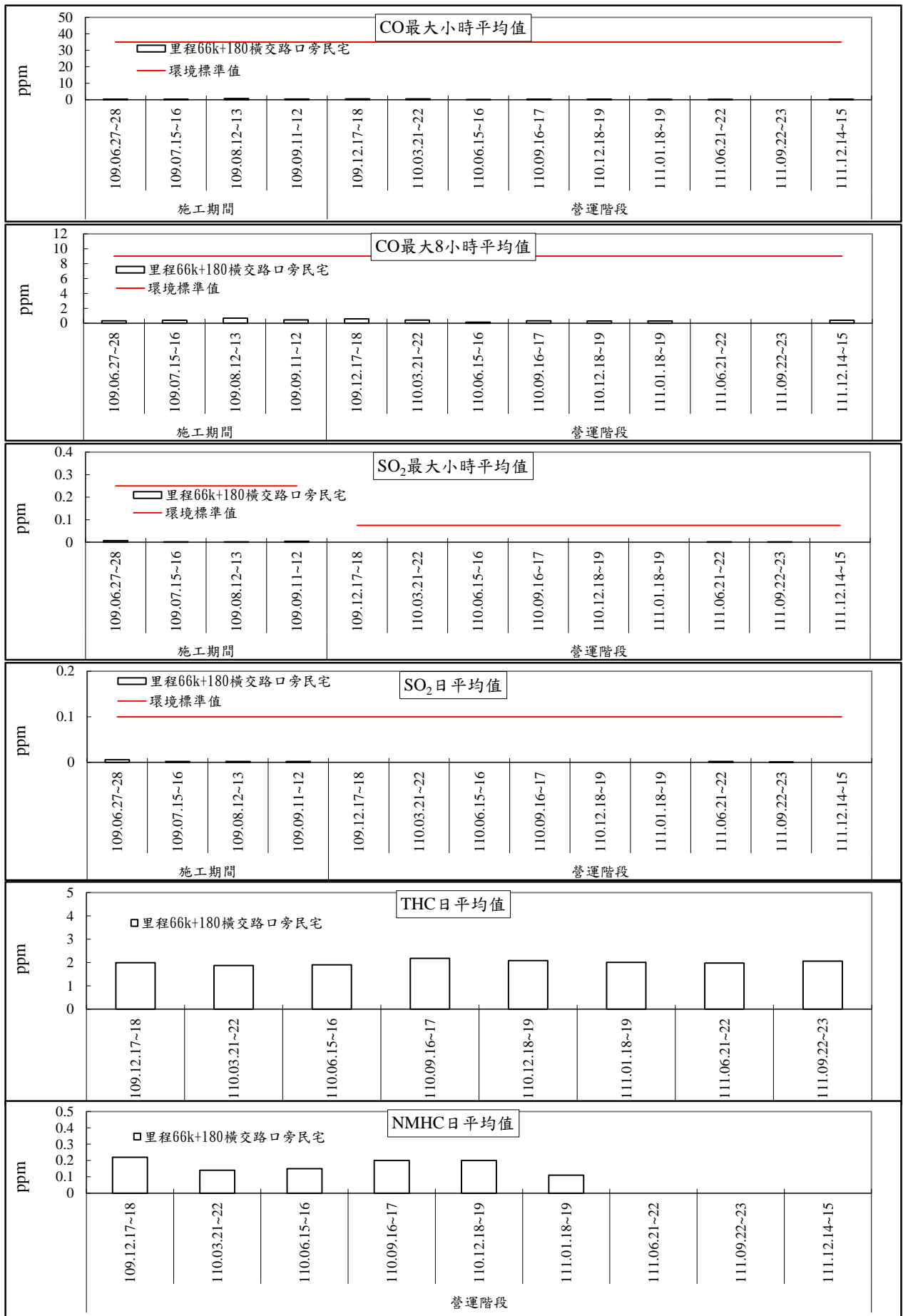
圖 2.8-2 里程 66k+180 橫交路口旁民宅空氣品質監測成果趨勢圖(2/2)
