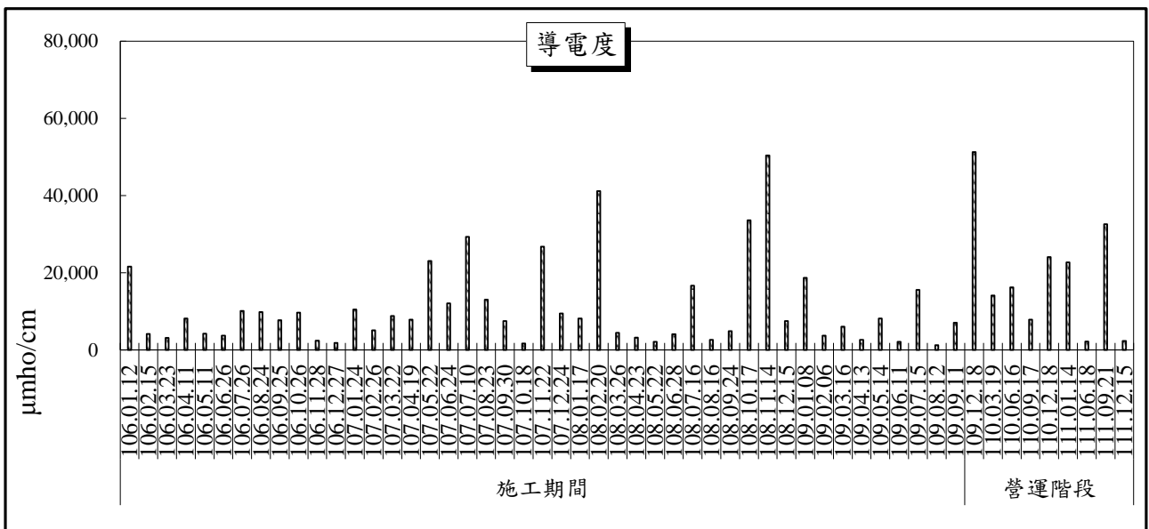
圖 2.10-2 池和橋監測結果變化趨勢圖(3/3)
