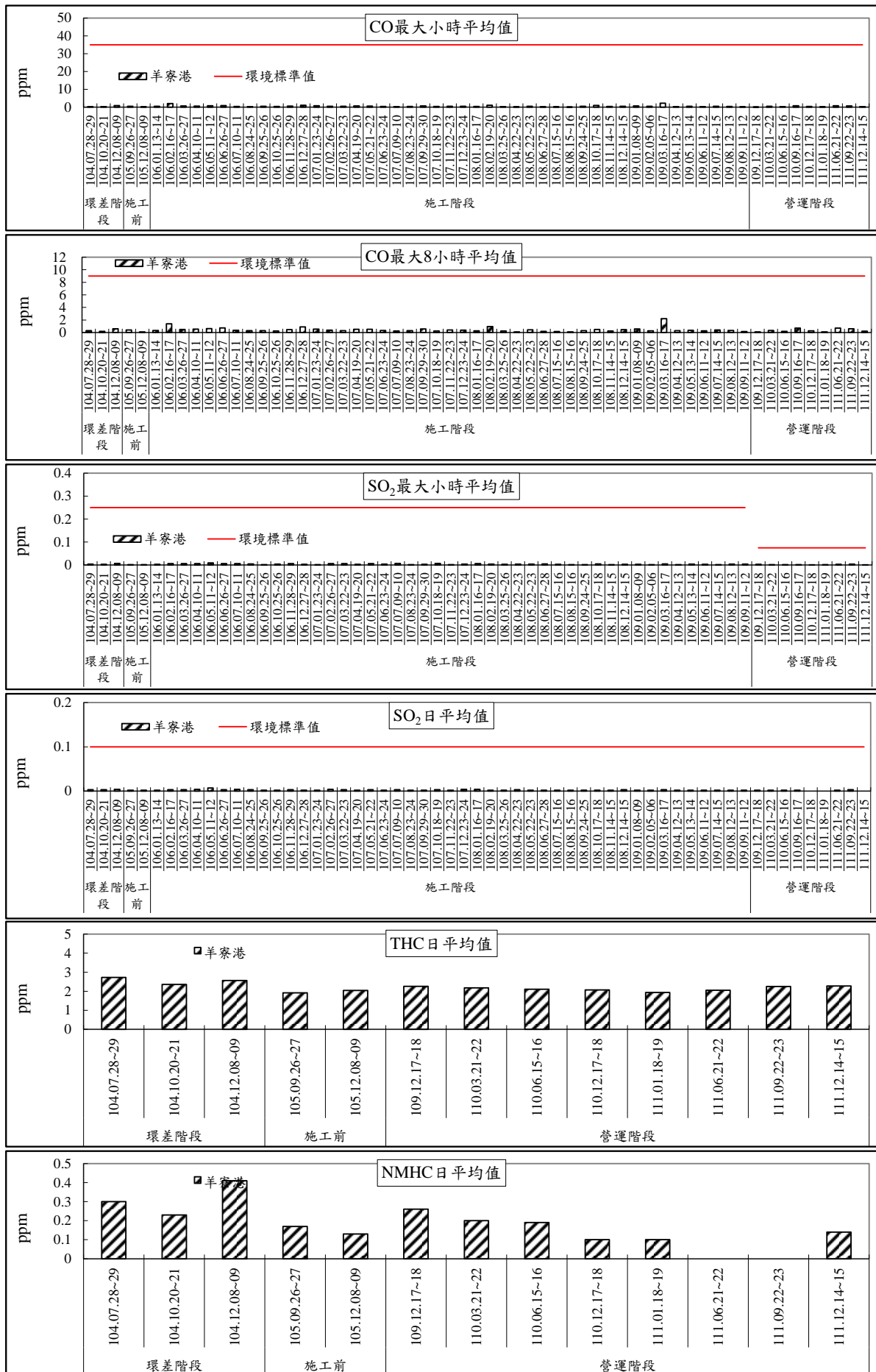
圖 2.8-1 羊寮港空氣品質監測成果趨勢圖(2/2)
