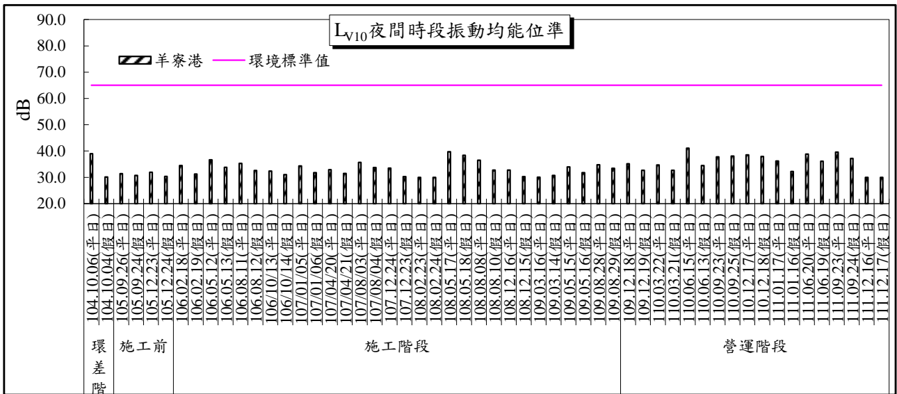
圖 2.9-2 羊寮港測站振動監測結果變化趨勢圖
