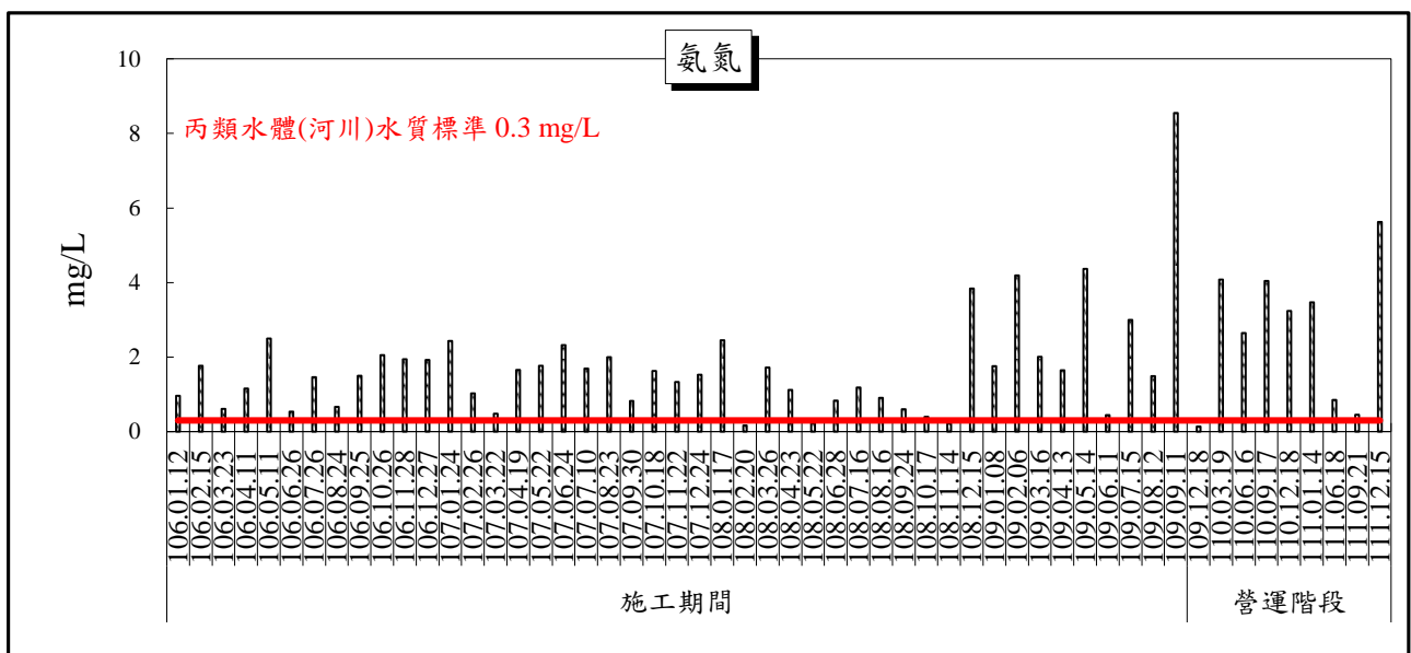
圖 2.10-2 池和橋監測結果變化趨勢圖(2/3)
