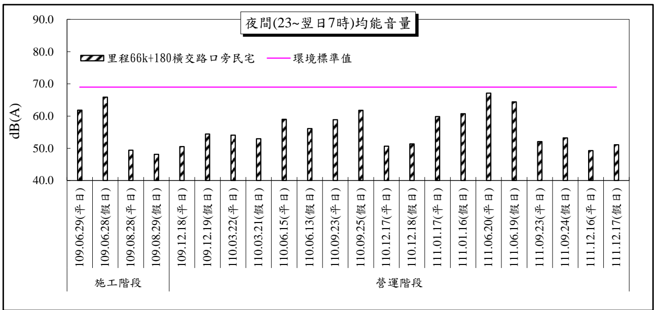
圖 2.9-3 里程 66k+180 橫交路口旁民宅測站噪音監測結果變化趨勢圖
