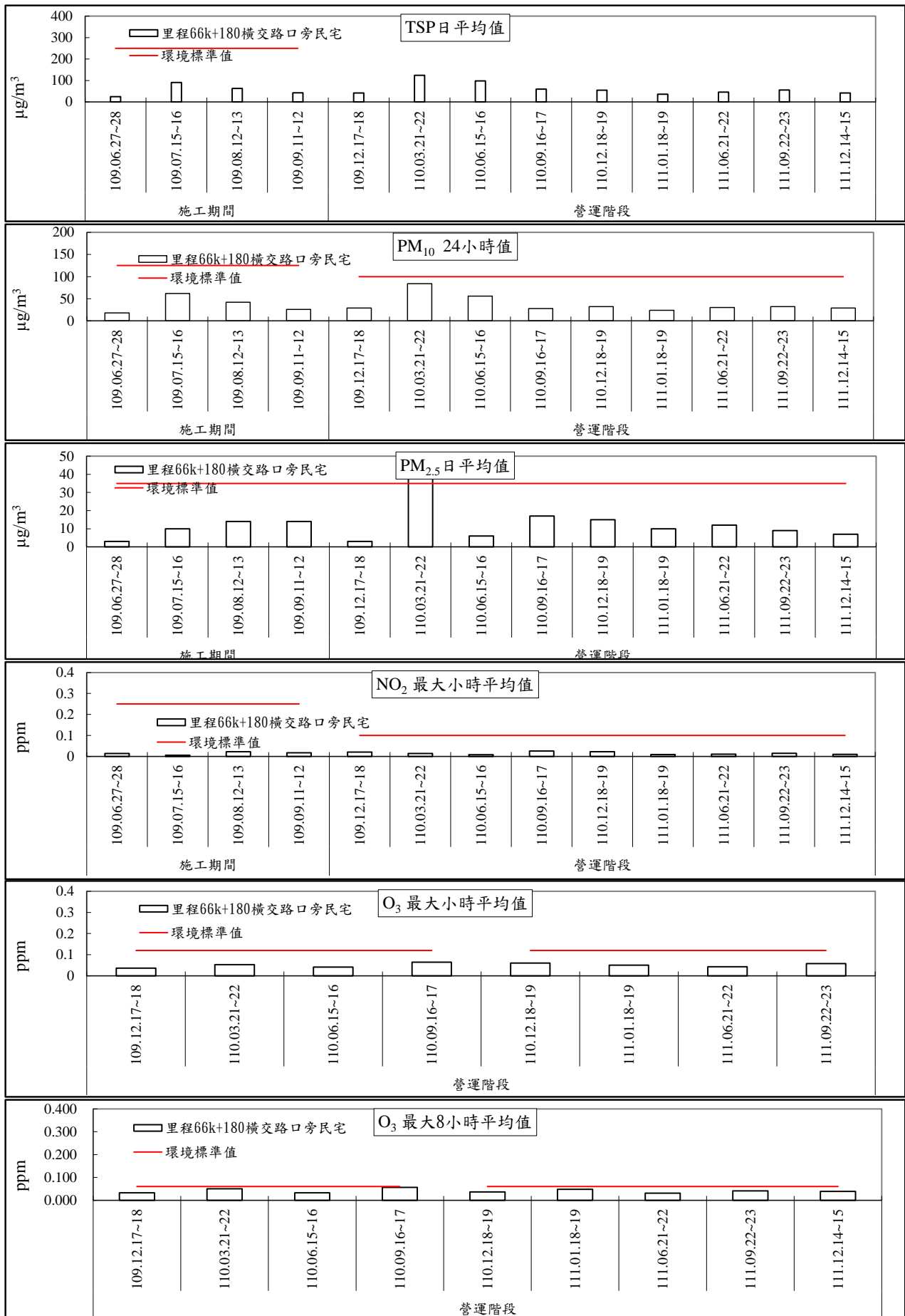
圖 2.8-2 里程 66k+180 橫交路口旁民宅空氣品質監測成果趨勢圖(1/2)
