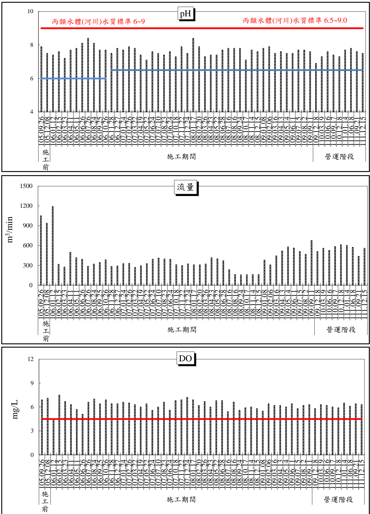
圖 2.10-1 新豐溪紅樹林橋監測結果變化趨勢圖(1/3)
