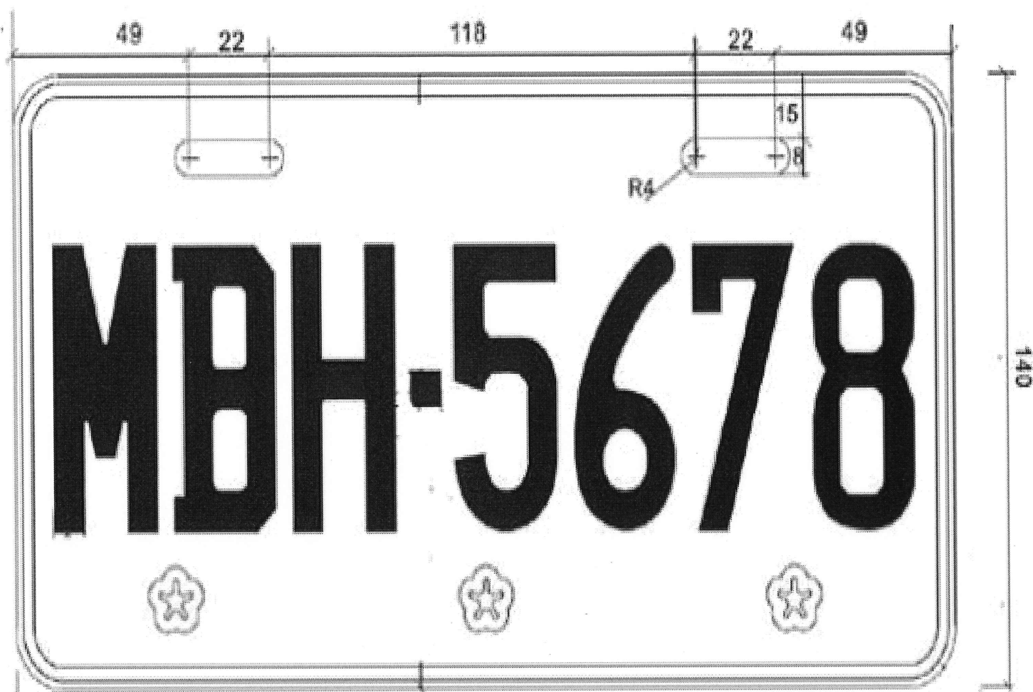
機車號牌(長260mm*高140mm)，螺絲鎖孔位置圖
